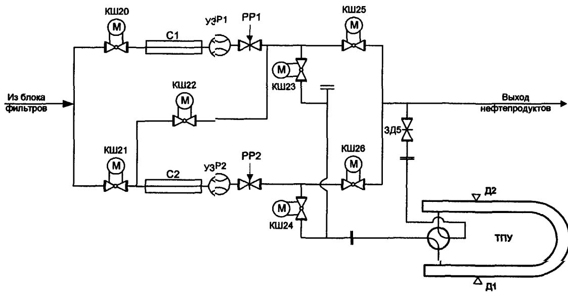
Рисунок Г.1 Принципиальная технологическая схема УУНП
