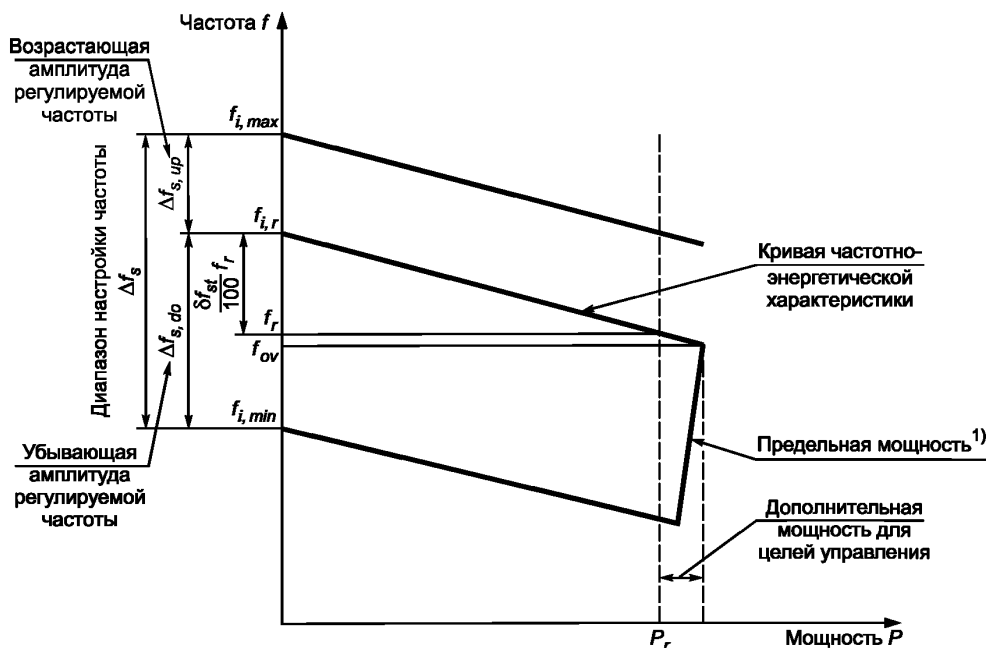
Рисунок 1 — Частотно-энергетическая характеристика диапазона регулируемой частоты
