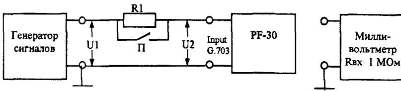
Рисунок 5. Измерение входного сопротивления прибора.
