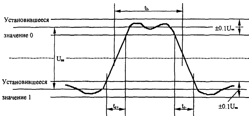
Рисунок 2в. Форма импульса для интерфейса V.36.
