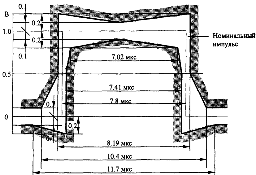
Рисунок 2а. Шаблоны импульсов для сонаправленного стыка (64 кбит/с).
