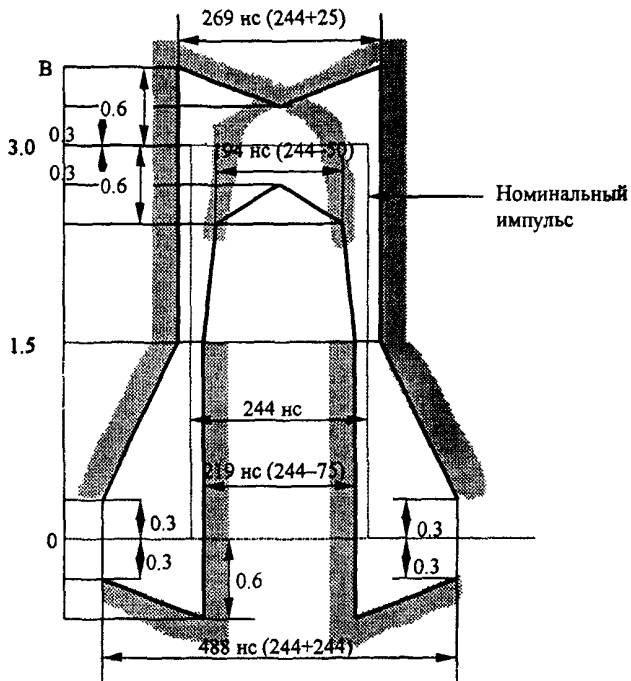
Рисунок 26. Шаблон импульса для первичного цифрового стыка (2 048 кбит/с).
