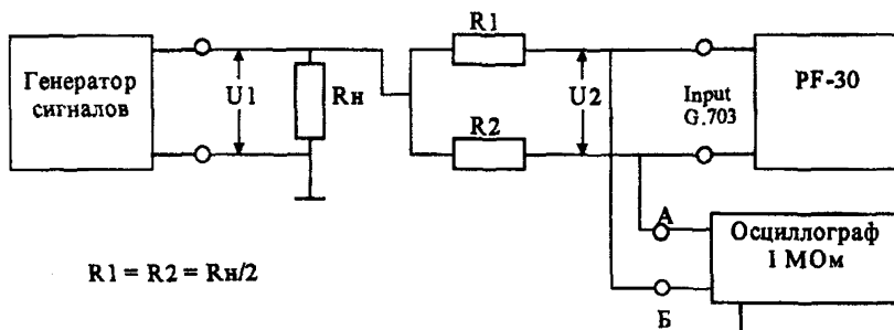
Рисунок 7. Измерение затухания асимметрии входа прибора
