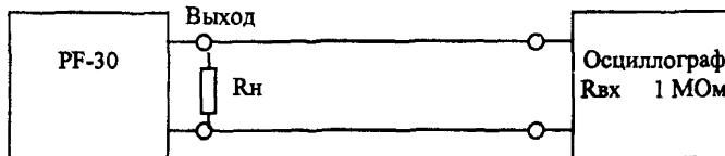
Рисунок 2. Схема для измерения параметров формы выходного сигнала.
