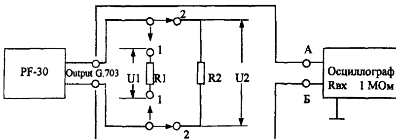
Рисунок 4. Схема измерения выходного сопротивления прибора
