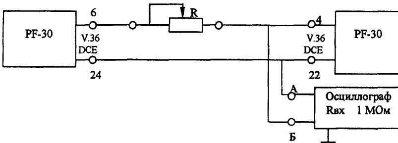
Рисунок 8б. Измерение чувствительности приемника на входе V.36 DCE
