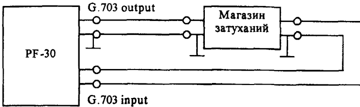
Рисунок 8а. Измерение чувствительности приемника на входе G.703
