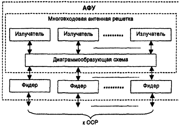
Рисунок А.4 - Построение АФУ на основе приемопередающей многоходовой антенной решеткой
