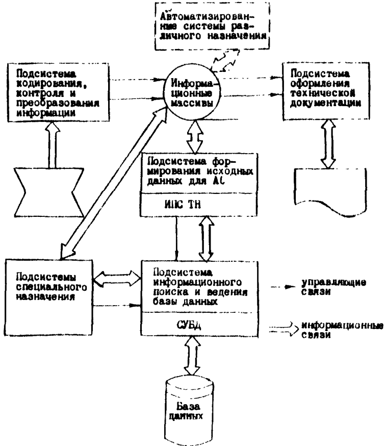
Схема взаимосвязей подсистем общего назначения
