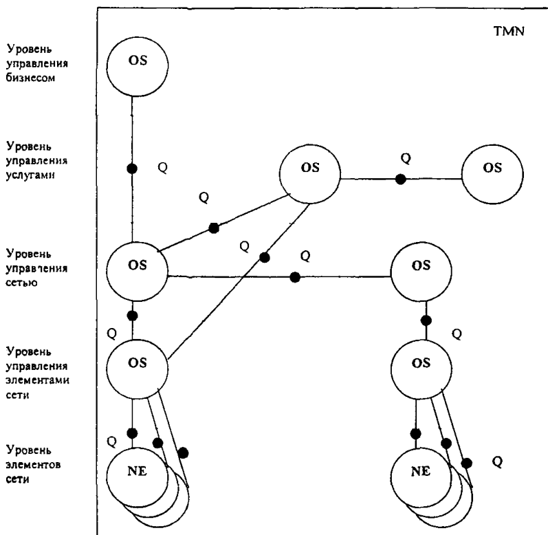
Рисунок 6 – Схема взаимодействия между OS и OS в пределах одной TMN
