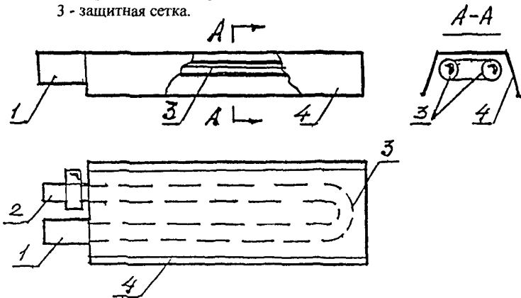
Рис. 1б. Схема “темного” газового инфракрасного излучателя
