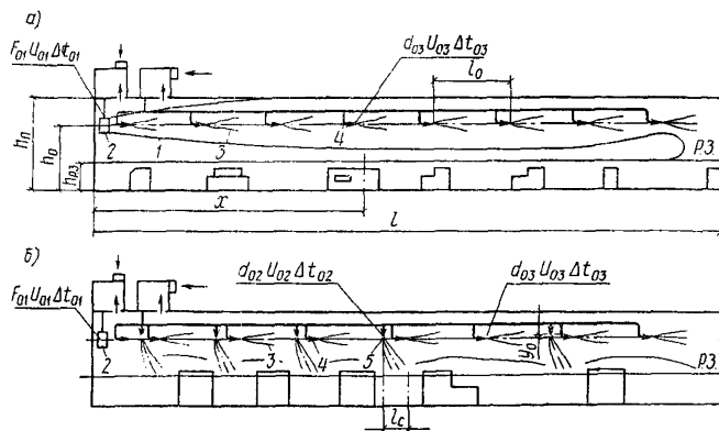
Рис. 1. Отопительно-вентиляционная система с направляющими соплами а - горизонтальными; б - горизонтальными и вертикальными
