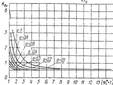
Рис.8. График для определения коэффициентов K_{в3} и K_c .
