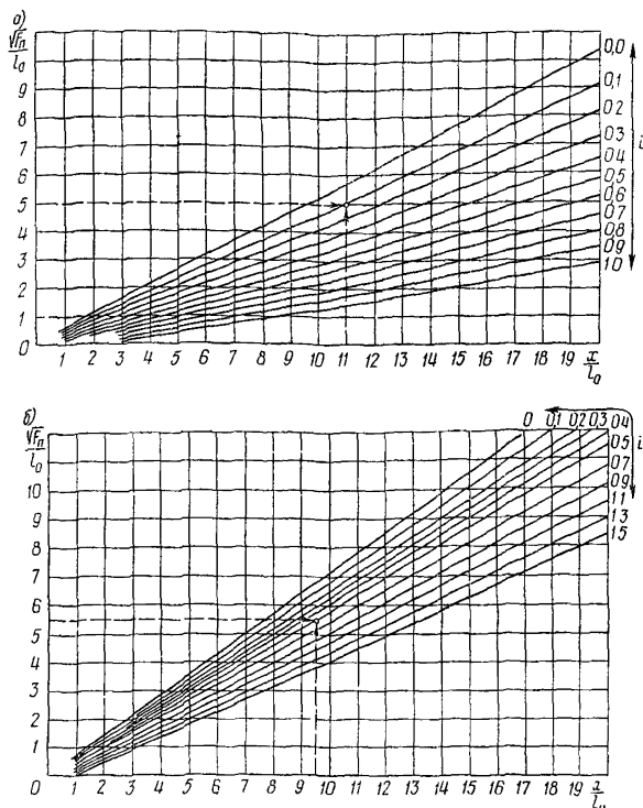
Рис.4. Номограмма для определения параметра i а - при m_1 = 6,2 ; m_2 = 6,2 ; m_3 = 4,5 ; б - при m_1 = 6,2 ; m_2 = 6,2 ; m_3 = 6,2
