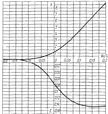
Рис.7. График для определения параметров А и Е
