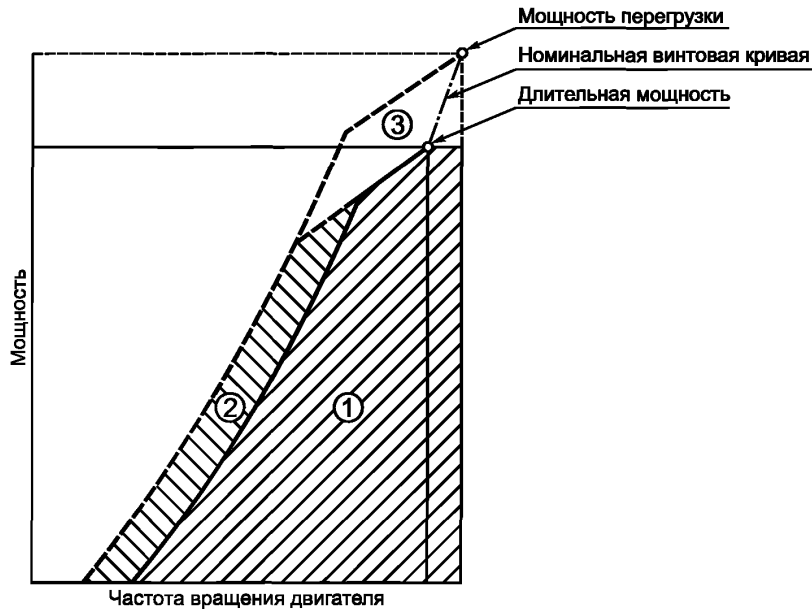
Рисунок 3 — Диаграмма «мощность — частота вращения»
