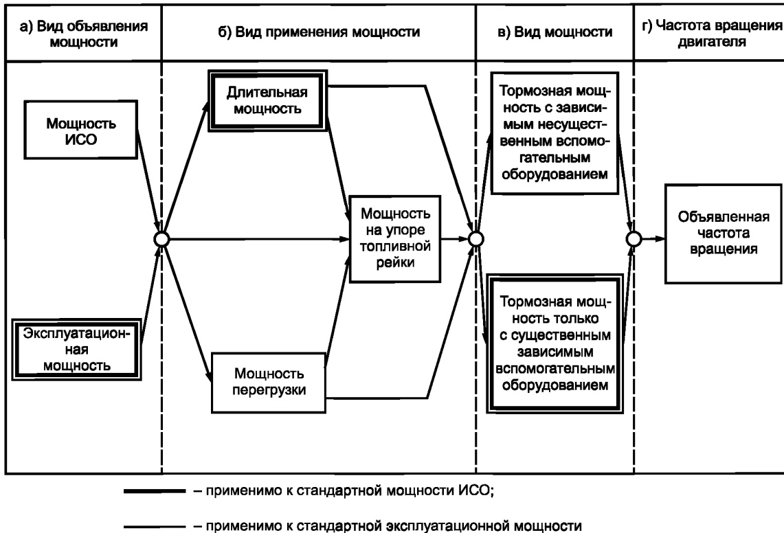
Рисунок 1 — Диаграмма, показывающая способы определения вида мощности
