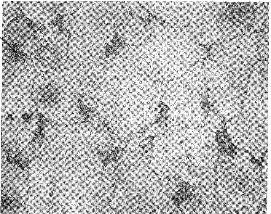
Рис. 12. Сплав М18. Начальная стадия пережога, слабая степень (температура закалки 530°С). Травление в реактиве № 2: а — \times 100 ; б — \times 500
