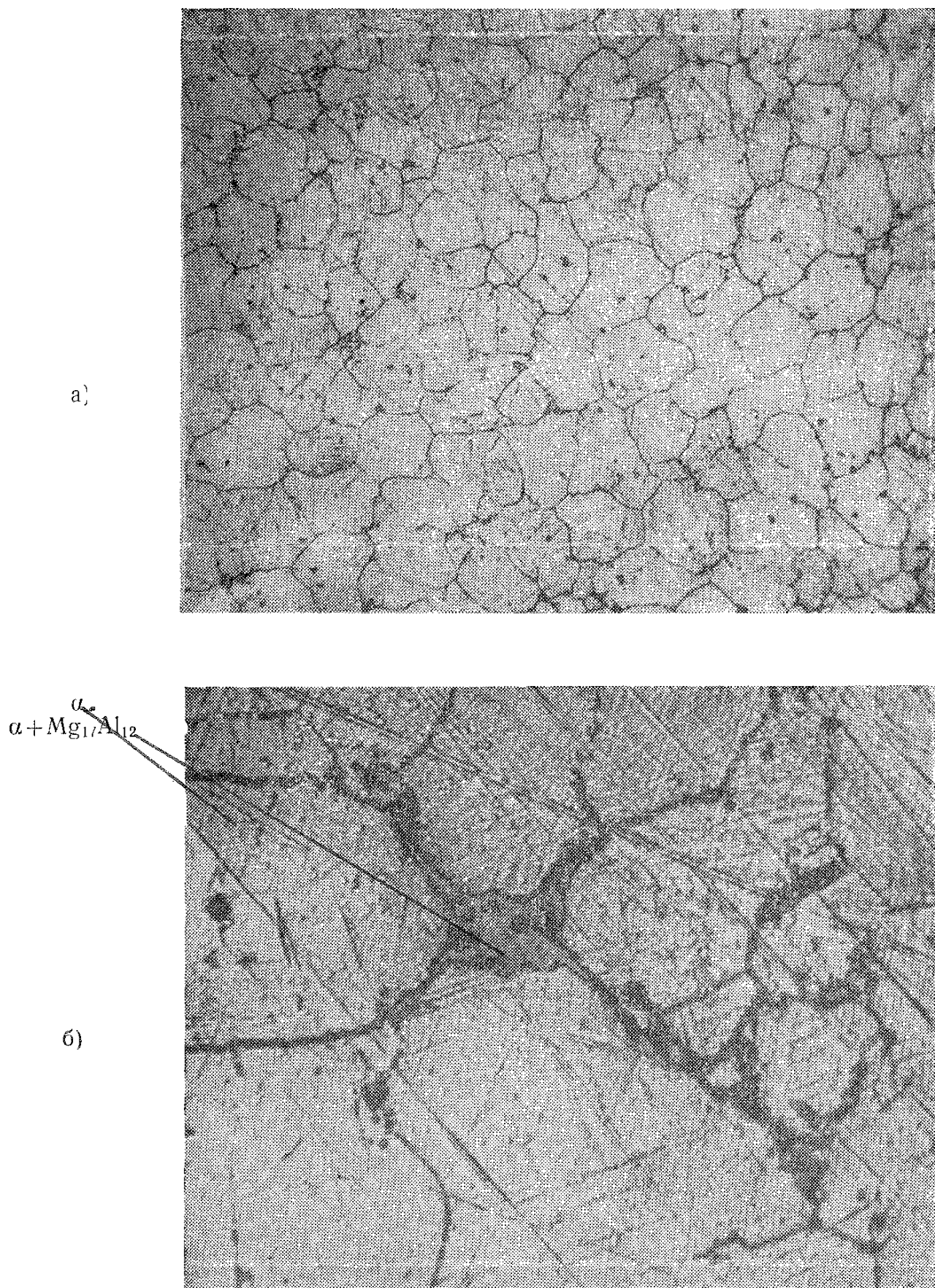
Рис 8 Сплав МЛ5, МЛ5пч, МЛ5он. Неполная закалка (температура закалки 415°C, время 4 ч). Травление в реактиве № 1. а — \times 100 ; б — \times 500
