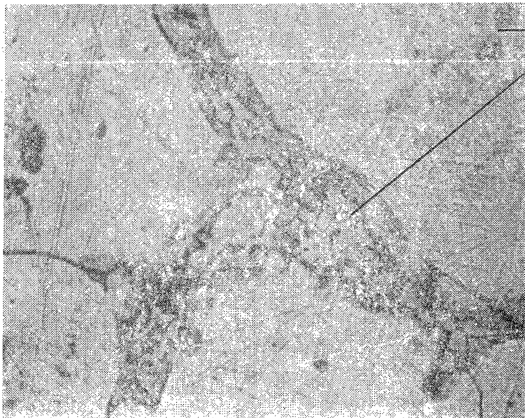
Рис. 5. Сплав МЛ5, МЛ5пч, МЛ5ол. Персеченный при закалке (температура закалки 500°С): а — ×160; б — ×500
