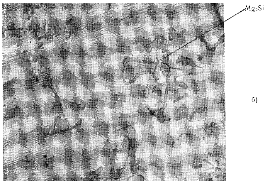
Рис. 3 Сплав МЛ5, МЛ5пч, МЛ5оп. Состояние Т4 (Закаленные) а — травление в реактиве № 1, \times 200 ; б — без травления, \times 500
