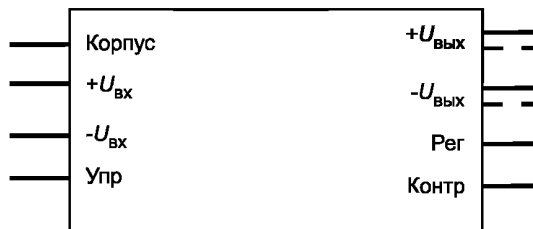
Рисунок Б.1 — Расположение выводов одноканальных СЭМ
