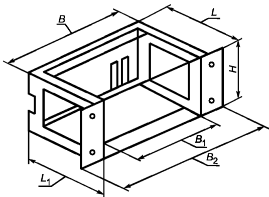
Рисунок 3 — Размеры корпусов СЭМ 2
