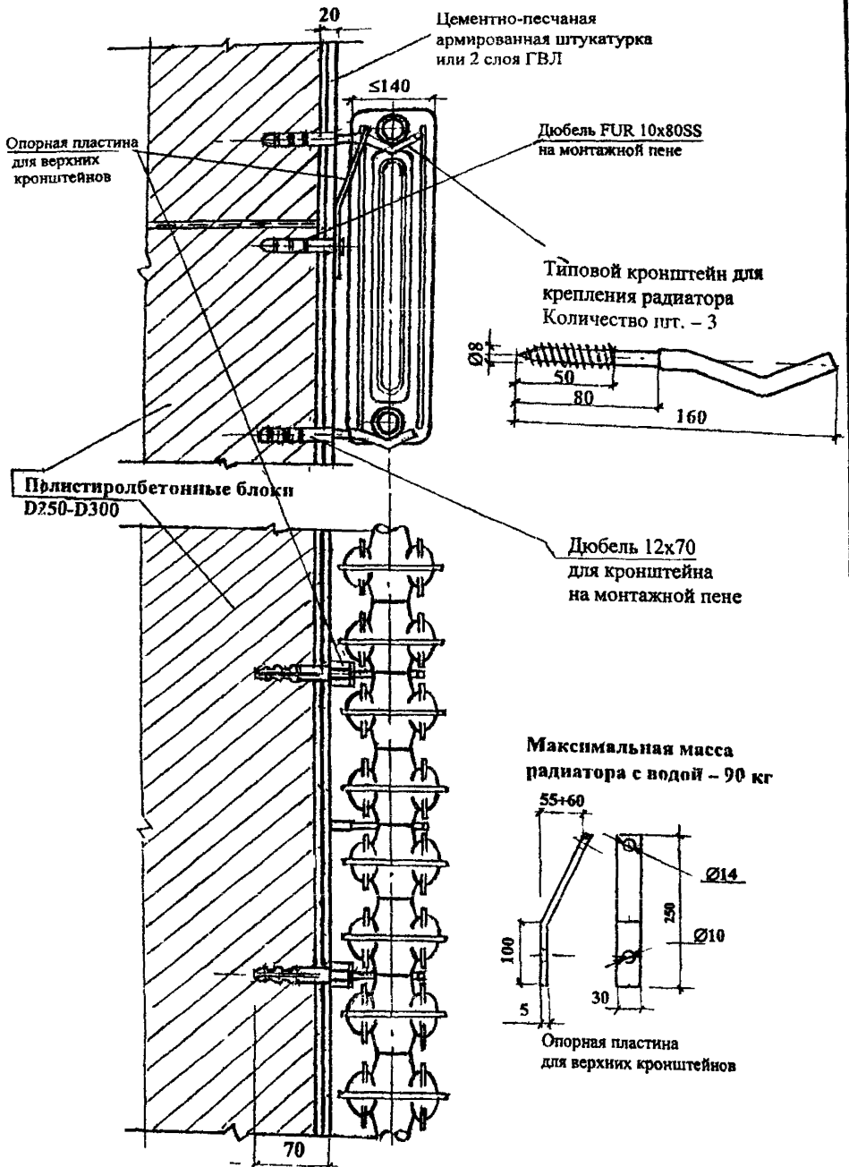
Вариант крепления чугунного радиатора
