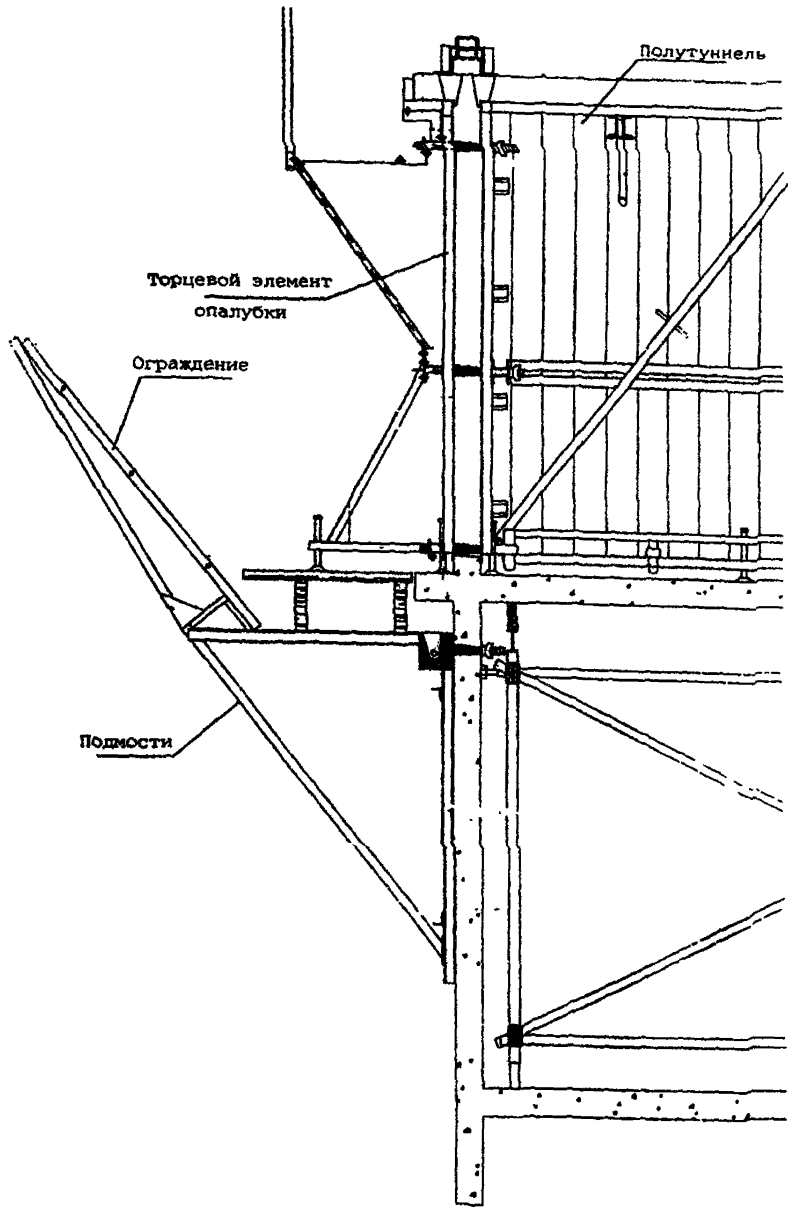
Разрез 2-2
