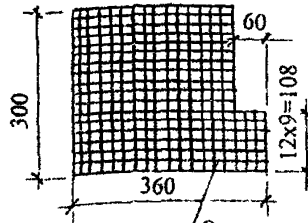
Оцинкованная сетка из проволоки Ø1,2 мм с ячейкой 12x12 мм по ГОСТ 3826-82
