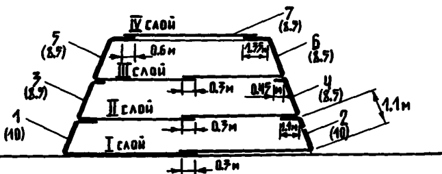
Рис.10. Схема расположения полотен:
