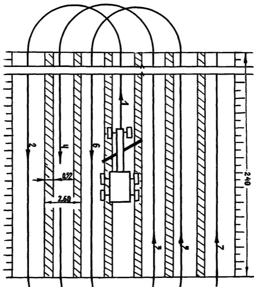
Рис. 3. Схема работы автогрейдера Д-557 при планировке: 1-7 - номера проходов
