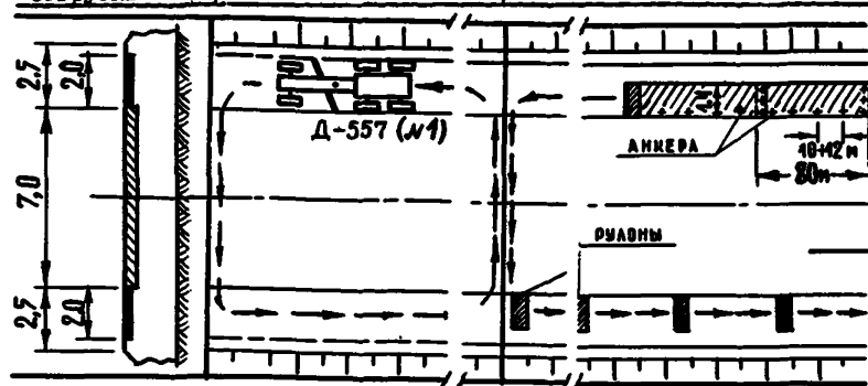
Рис.8. Схема потока по укреплению обочин с
