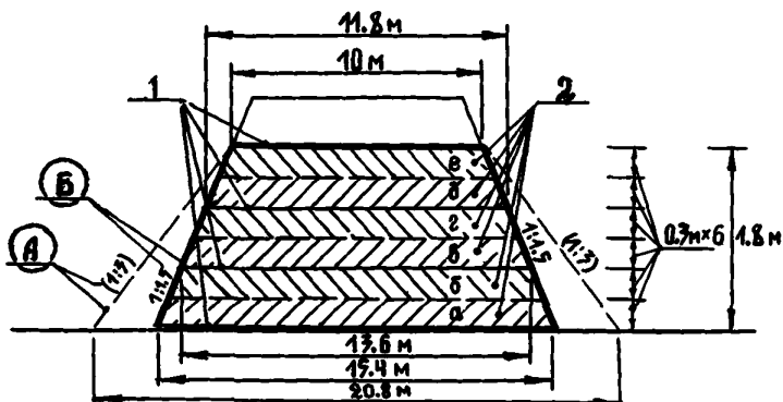
Рис.9. Поперечный профиль насыпи, отсыпаемой из переувлажненных грунтов:
