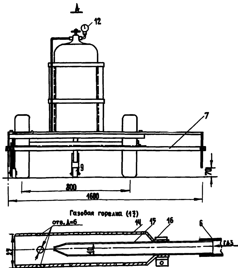
Рис. 12. Схема установки для соединения полотен синтетических материалов: 1—рама тележки; 2—колесный ход; 3—газовый баллон; с редуктором; 4—установочный каркас; 5—газопровод (металлическая трубка); 6—газопровод (гибкий напорный шланг на 1,5 атм); 7—поддерживающий валик; 8—опора горелки; 9—колесо опоры горелки; 10—нижнее свариваемое полотно; 11—верхнее свариваемое полотно; 12—манометр; 13—газовая горелка; 14—внешняя защитная металлическая трубка с отверстиями; 15—трубка газопровода; 16—хомут
