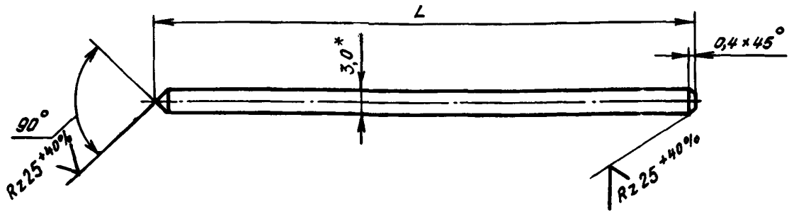
Размеры, мм
