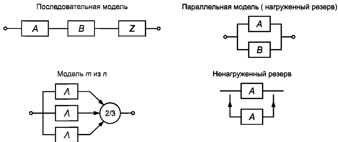
Рисунок A.5 — RBD для независимых блоков
