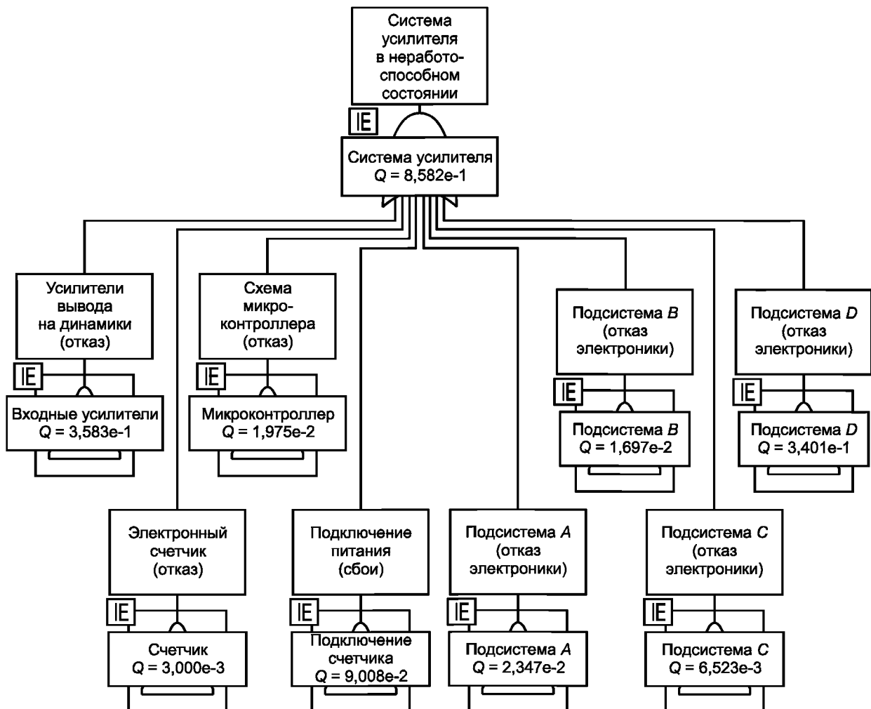
Рисунок А.2 — Дерево неисправностей для аудиоусилителя
