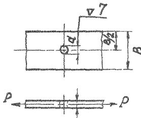
Фиг. 3 Форма и размеры рабочей части образца с симметрично расположенным поперечным отверстием
