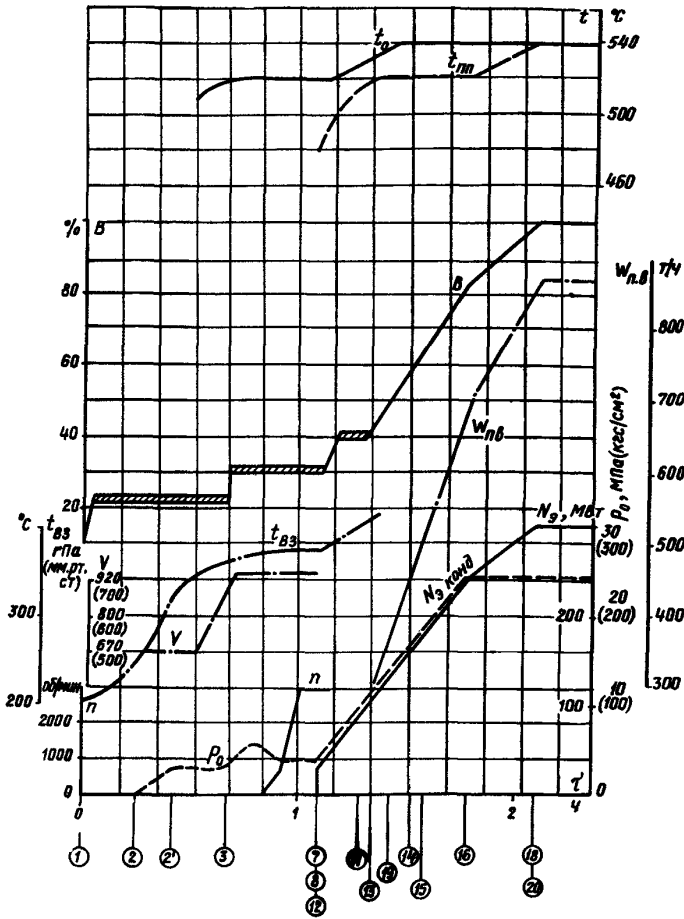
Рис. 8. График-задание пуска блока из горячего состояния (температура паровпуска ЦВД 400°C, температура паровпуска ЦСД ≥ 420°C, продолжительность простоя 2-8 ч)
