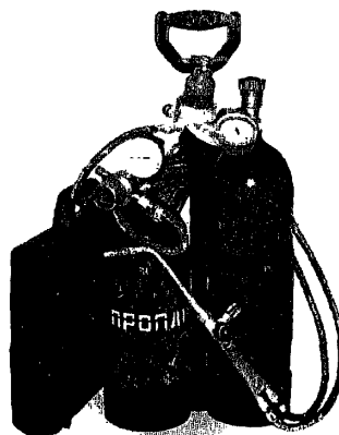
На снимке: пропановый пост малой мощности ПГС-4/5-001П с 4-литровым пропановым и 5-литровым кислородным баллонами.
