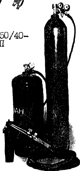
На снимке: пропановый пост малой мощности ПГС-4/5-001П с 4-литровым пропановым и 5-литровым кислородным баллонами.
