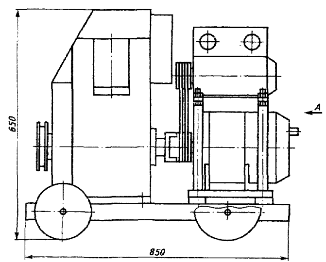
Общий вид и габаритные размеры агрегатов „ОСА-300-2 Комби” и „ОСА-300-4 Комби”
