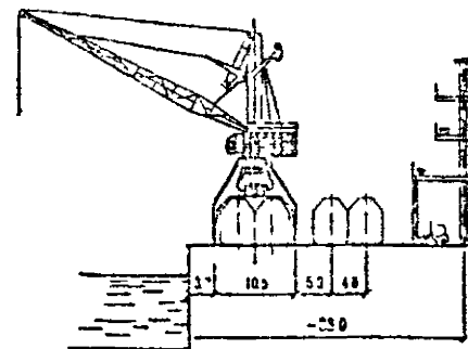
Вариант с четырьмя прикрановыми железнодорожными путями
