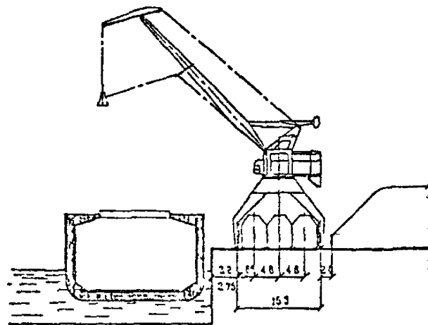
Вариант с тремя прикрановыми железнодорожными путями
