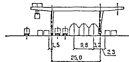
Вариант с 3-мя железнодорожными путями на грузовом фронте
