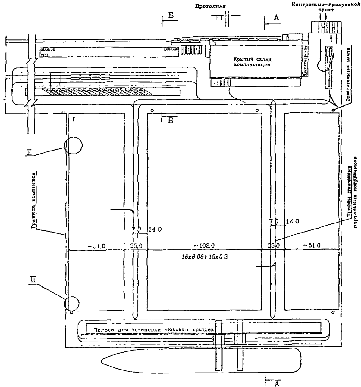
Рис.3 Схема механизации N1 с порталными погрузчиками и размещением контейнеров параллельно линии кордона. План.
