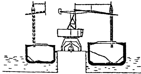
Механический перегружатель на портале
