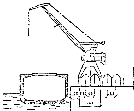
Вариант с четырьмя прикормонными железнодорожными путями
