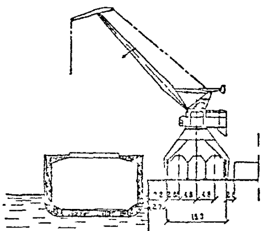
Вариант с тремя прикормонными железнодорожными путями
