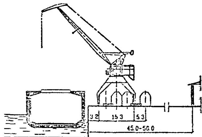
Вариант с тремя прикромными железнодорожными путями
