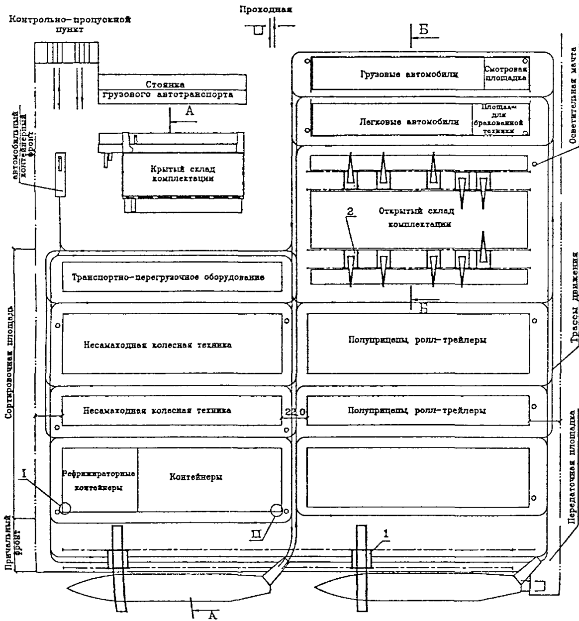
Рис. 5 Схема механизации НЗ с использованием порталых погрузчиков
