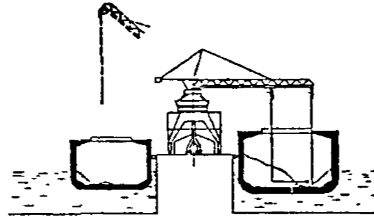
пневматический перегружатель на портале
