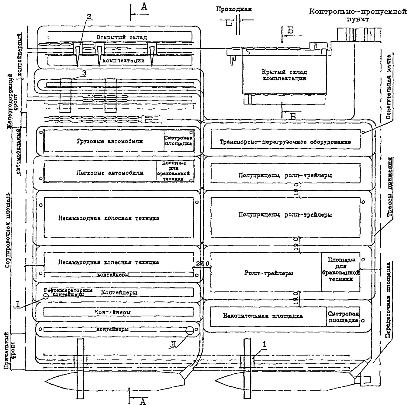
Рис.1 Схема механизации N1 с использованием тягачей с полуприцепами. План
