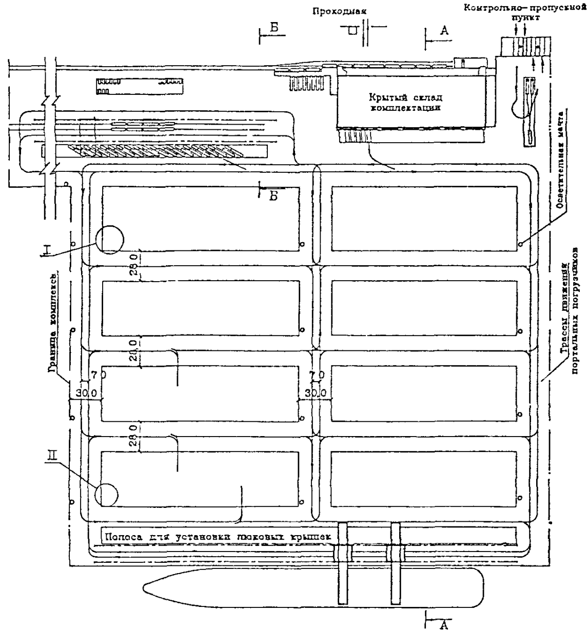
Рис. 1 Схема механизации N1 с порталными погрузчиками и размещением контейнеров перпендикулярно линии жордонж. П. III
