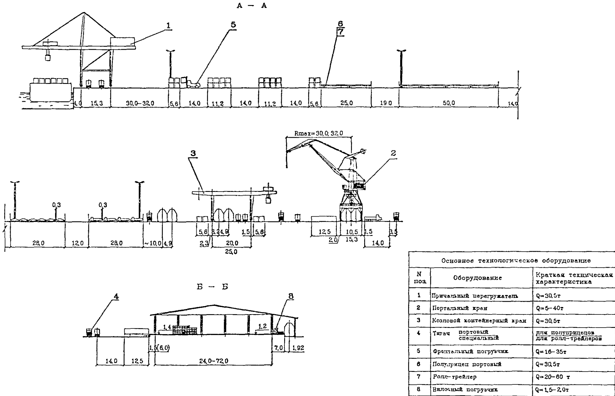
Рис.2 Схема механизации N1 с использованием тягачей с полуприцепами. Разрезы
