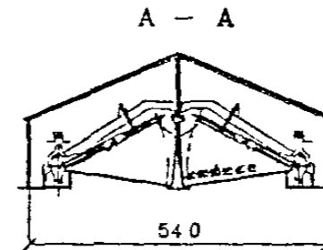
загрузка и разгрузка комбинированным полупортальным краном
