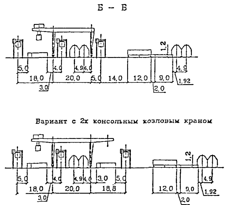
Рис. 4 Схема механизации №1 с портальными погрузчиками и размещением контейнеров параллельно линии кордона Разрезы
