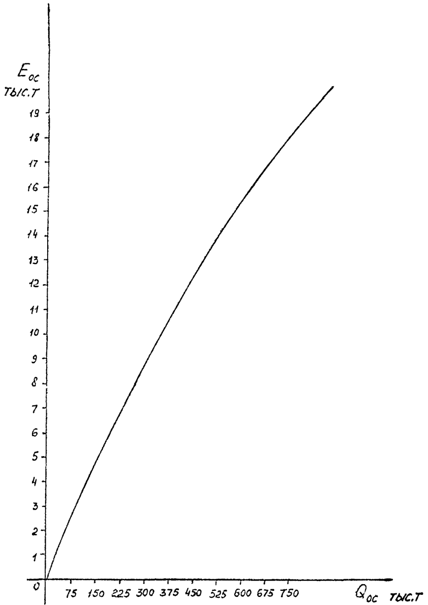
Рис. 18. Зависимость потребной вместимости открытого склада от грузооборота
