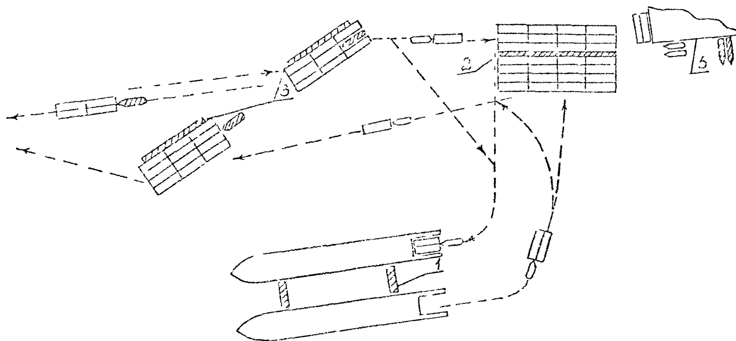
Функционирование лихтерового комплекса по схеме 1
