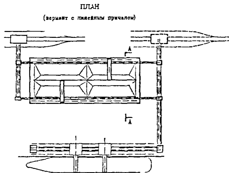
элеваторно-конвейерный перегружатель
