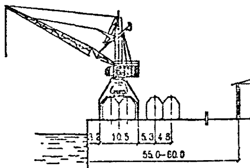
Вариант с 4-мя прикромными железнодорожными путями
