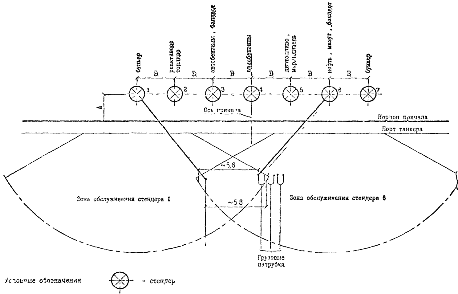
Рис.20 Схема совмещения зон обслуживания стеньгеров с зоной расположения судовых приемно-отливных патрубков
