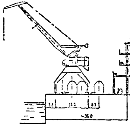
Вариант с тремя прикрановыми железнодорожными путями
