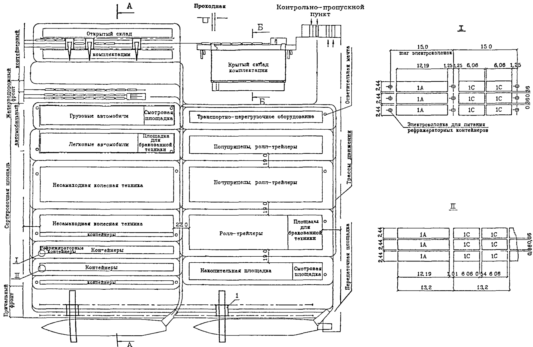
Рис.3 Схема механизации №2 с использованием фронтальных погрузчиков План
