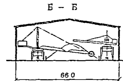
загрузка-стакером разгрузка-реклаймером
