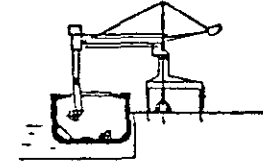
роторно-конвейерный перегружатель (элеваторно-конвейерный скребково-конвейерный)
