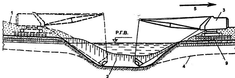
Схема 4 - экскаватор-драглайном со сланей
