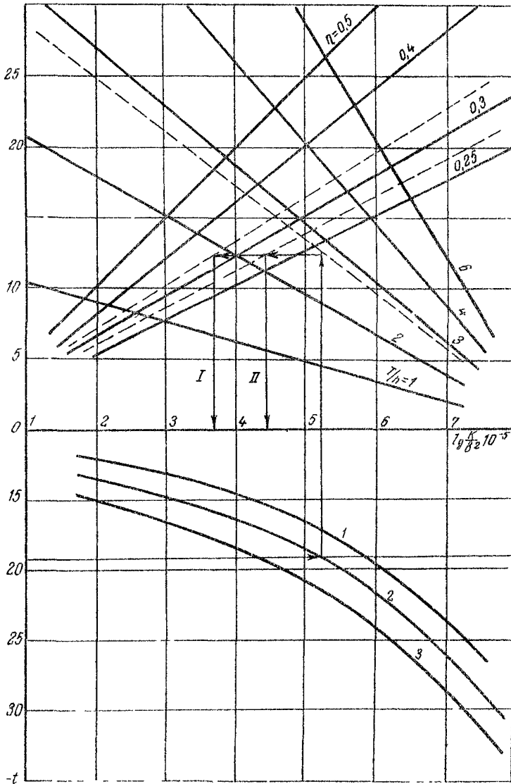
Рис. 5. Номограмма для определения допустимого лучения дорожных одежд нежесткого типа Асфальтобетонное покрытие на битумах марок: 1 - БНД 40/10; 2 - БНД 60/90; 3 - БНД 90/130
