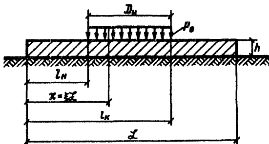
Рис.2. Расчетная схема балки на упругом основании, нагруженной симметрично в середине, для расчета на растяжение при изгибе
