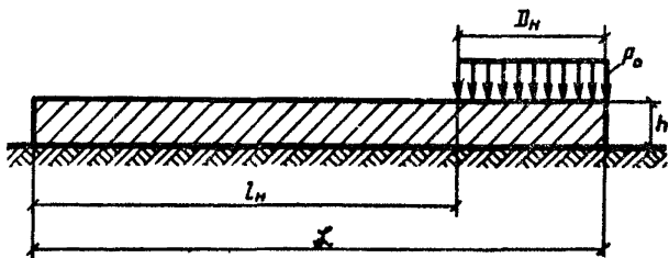
Рис.1. Расчетная схема балки на упругом основании, нагруженной на конце, для расчета по сдвигу устойчивости в грунте основания
