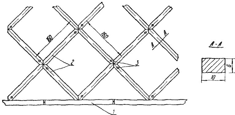
Рис. 3. Облегченная решетчатая конструкция с диагональным расположением элементов:
