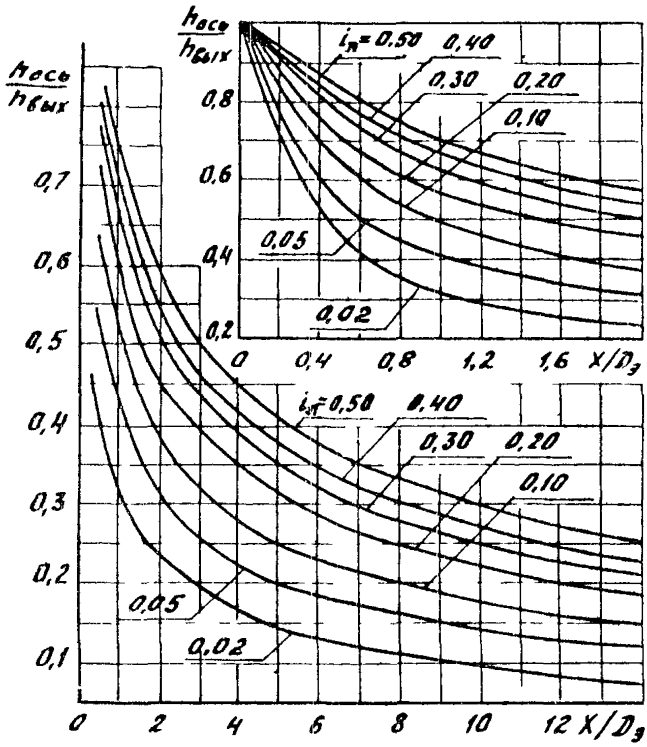
Рис. 4. График для определения глубин по оси потока h_{\text{ось}} на укреплении
