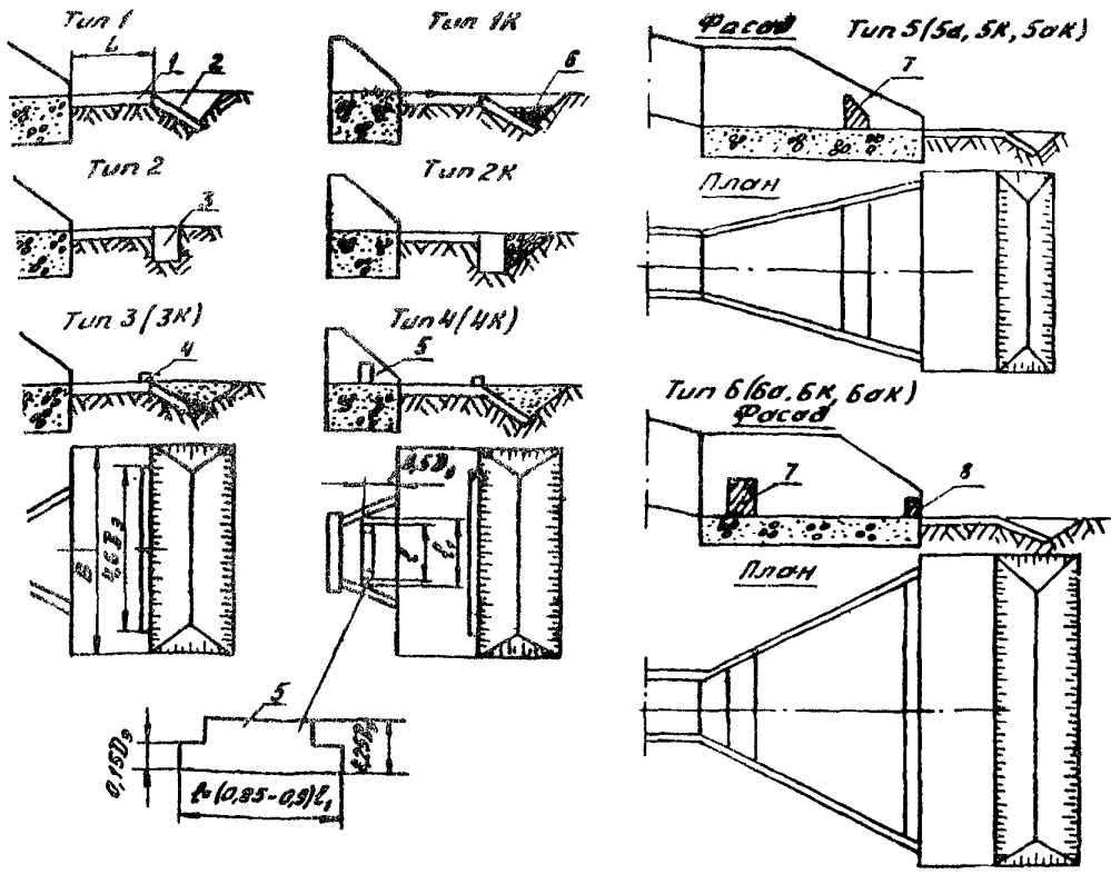
Рис. 6. Типы выходных русл: 1 - репление; 2 - предохранительный откос; 3 - вертикальная стенка; 4 - в конце укрепления; 5 - стенка в раструбе; 6 - каменная наброска; 7 - стенка в расширяющемся раструбе; 8 - стенка на выходе из расширяющегося раструба
