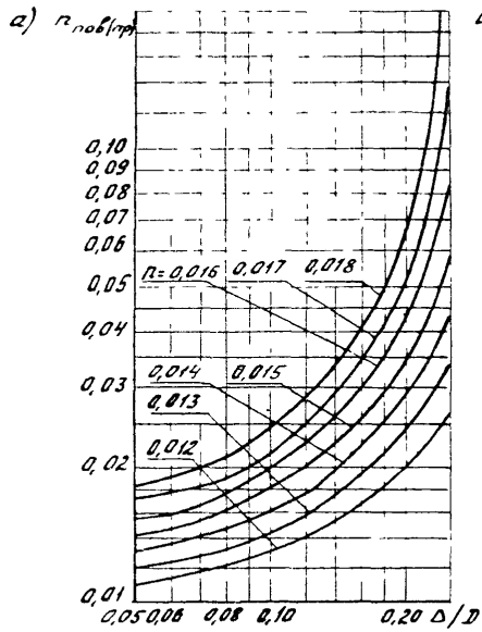
Рис.2. График для определения коэффициента приведенной повышенной шероховатости в круглых трубах: а - \eta_{пов}(пр) = f(\Delta/D) при h/D \geq 0,225 ; б - поправочный коэффициент K_h = f(h/D)
