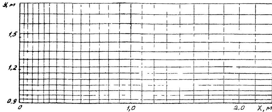
Рис. 1. Вариант неравномерной разностной сетки для расчета растекания потока в ложе с прямолинейными боковыми стенками (в силу симметрии области течения относительно оси трубы сетка построена для половины области)
