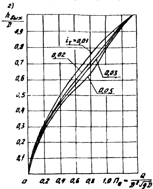
Рис. 1. График для определения глубин на выходе из труб: а - круглых; б - прямоугольных, работающих при \Pi_a > 0,8 при полунапорном режиме; в - овальных; г - гофрированных с учетом их возможной "зарядки"
