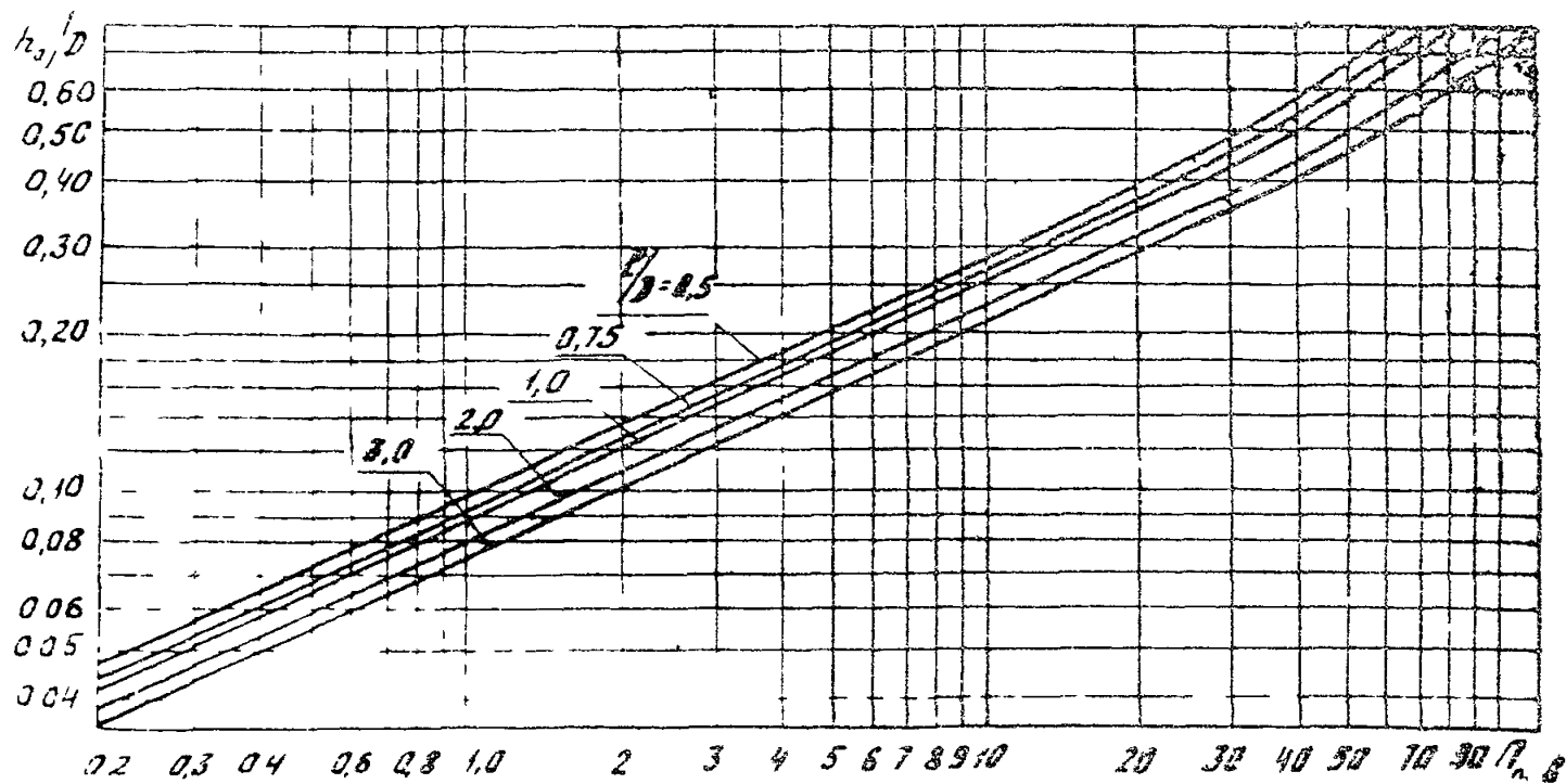
Рис. 1. График для определения нормальных глубин h_0 в круглых трубах при ступенчатой укладке авеньев
