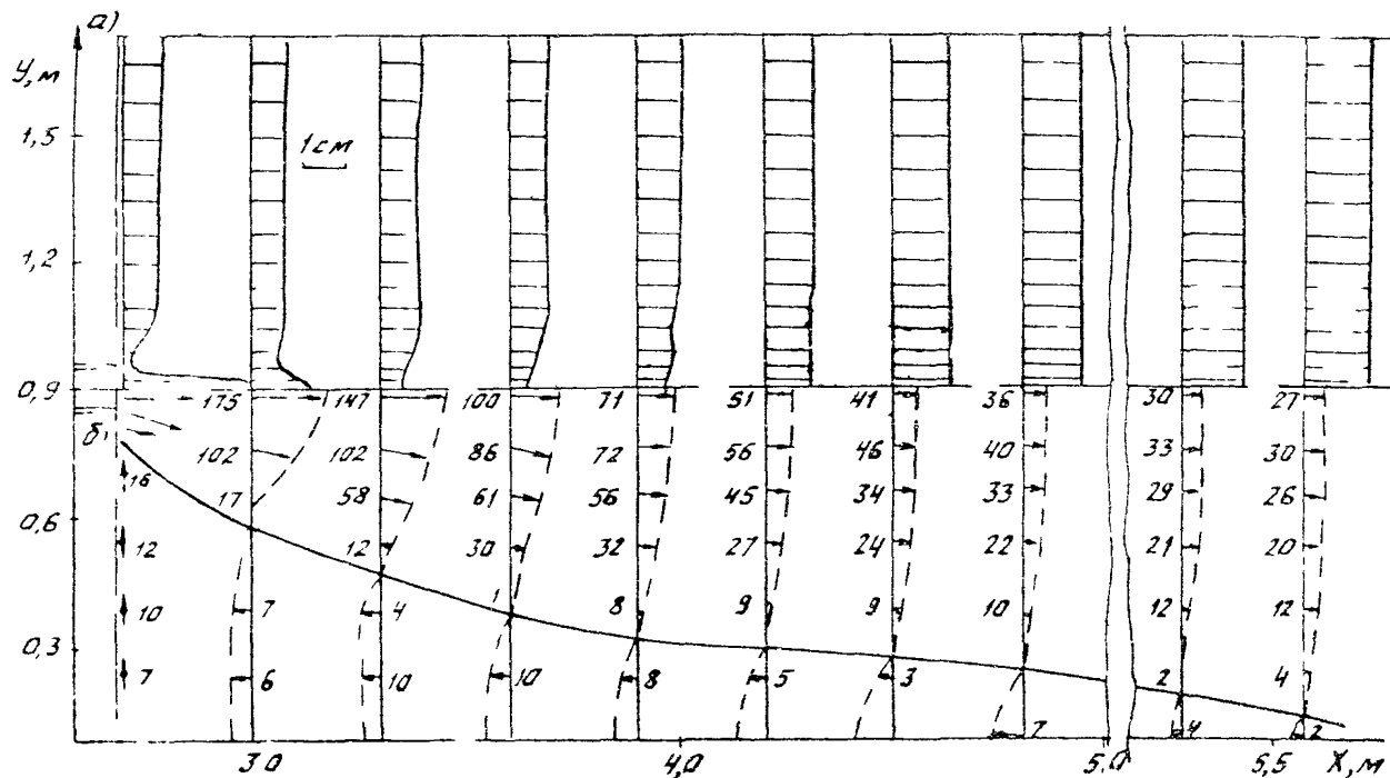
Рис. 3. Глубины (а) и скорости (б) потока при истечении его в лог с уклоном дна i_{\text{л}} = 0,001 (остальные параметры те же, что и на рис. 2): \vec{v} — векторы скорости, 7...175 — их абсолютные значения; — линия нулевых скоростей
