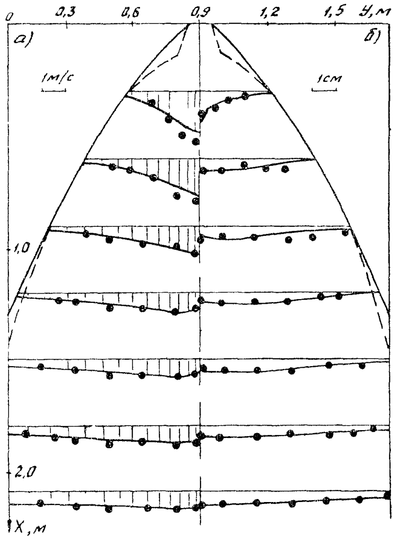
Рис. 2. Глубины и скорости потока при истечении его в лот шириной 1,8 м с плоским бетонным наклонным дном ( \lambda = 0,05 , \mu = 0,014 ) из круглой трубы диаметром D = 0,1 м, скоростью и глубиной на выходе V_{\text{вых}} = 1,78 м/с, h_{\text{вых}} = 0,035 м, приведенной шириной выхода B_{\text{вых}} = 0,064 м; а - эпюры скоростей; б - эпюры глубин, — — расчет, ••• - эксперимент; - - - границы растекания в эксперименте
