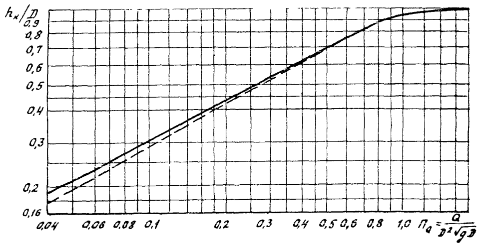
Рис. 2. График для определения критической глубины в трубах: — — — круг- лых; - - - - оvoidальных
