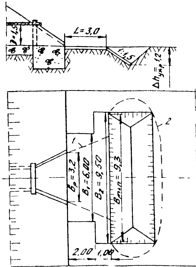
Рис. 1. Конструкция и размеры укреплений, полученные в результате расчета нижнего бьефа трубы при \tau_A < 0,02 : 1—граница растекания, 2—контур воронки размыва
