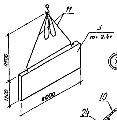
д) стропка цокольной стеновой панели
