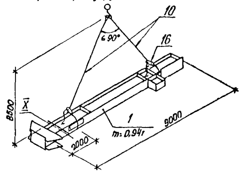
г) стропка подкрановых балок
