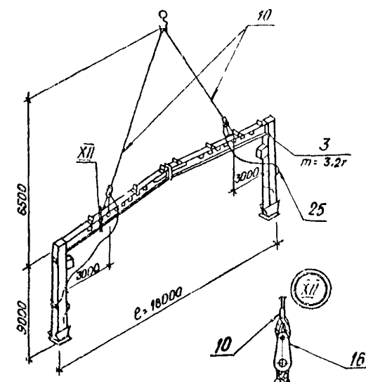
в) стропка рамы каркаса при монтаже
