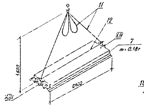
ж) кровельной панели ПКМ-120
