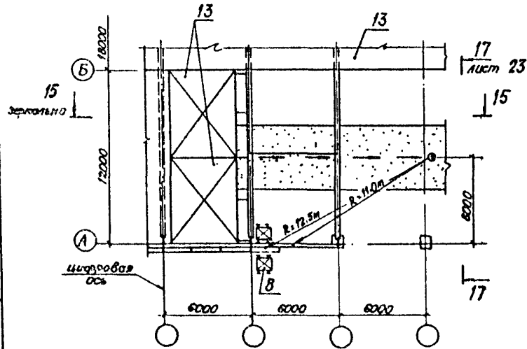
Схема монтажа стенового ограждения в пролете А-Б
