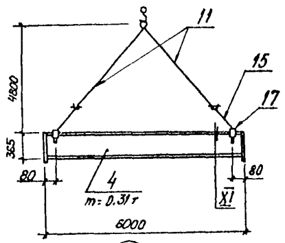
г) стропка подкрановых балок
