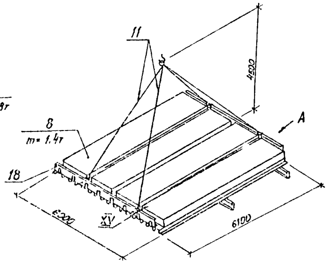
и) картин покрытия размером 6x6м
