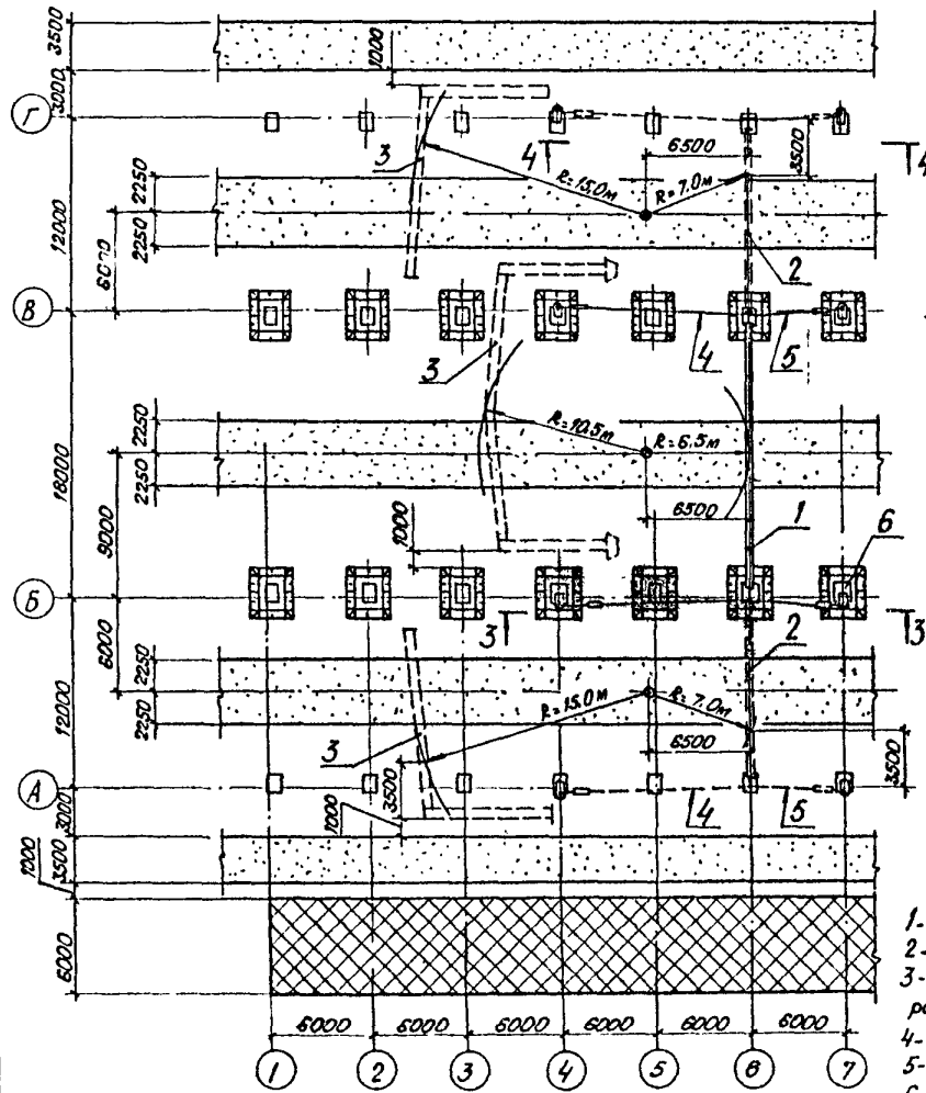
Схема монтажа первых рам и полурам по оси „б“
