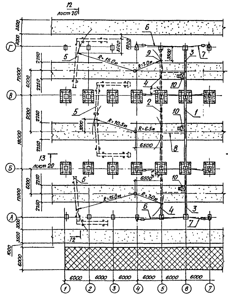
Схема монтажа второй рамы (полурамы) каркаса
