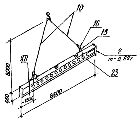
б) стропка балок рамы при укрупнительной сборке
