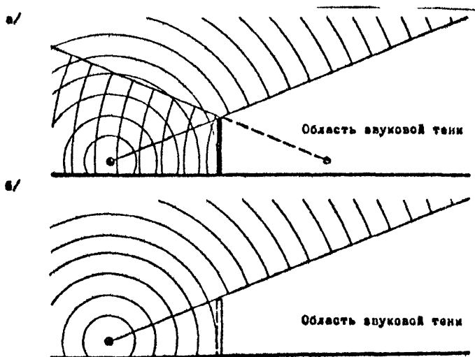
Рис.10.2. Образование звуковой тени: а - за шумоотражающим барьером; б - за шумопоглощающим барьером.
