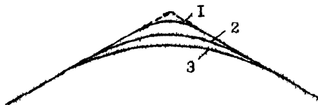
Рис.2.6. Уменьшение величины смещения кривой от вершины угла при разбивке закругления сопряженными переходными кривыми: 1 - круговая кривая малого радиуса; 2 - сопряженные переходные кривые; 3 - круговая кривая большого радиуса.
