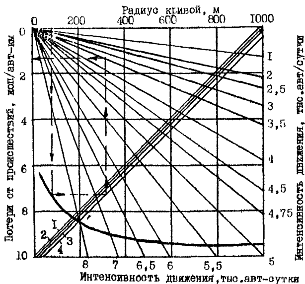
Рис. 9.5. Номограмма для определения потерь от дорожно-транспортных происшествий на кривых в плане при различной интенсивности /расстояние видимости: 1 - более 600 м; 2 - 300 м, 3 - 100 м/.
