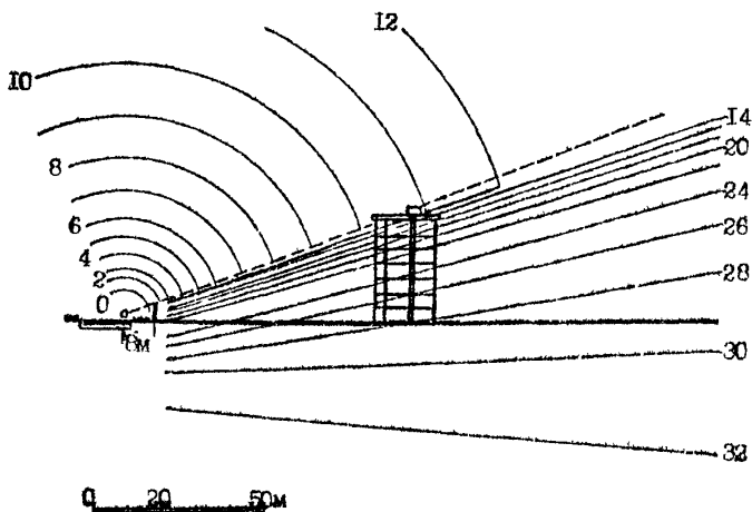
Рис.10.9. Применение прозрачного шаблона для определения снижения уровня звука за шумозащитным барьером при расстоянии от источника звука 8 м. Цифры обозначают относительное снижение уровня звука в дБА.
