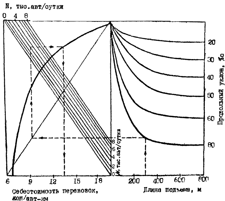
Рис.9.6.Номограмма для определения себестоимости перевозок на подъемах.
