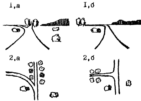
Рис. 2.3. Примеры неудачных примыканий дорог, создающие у водителей неправильное представление о дальнейшем направлении дороги: а - ложный ход; б - кажущийся поворот дороги; 1 - вид дороги; 2 - план дороги.
