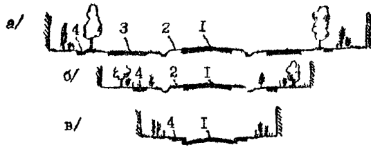
Рис.9.1. Поперечные профили дорог в малых населенных пунктах: а - дорога в насыпи при большой ширине улицы; б - то же при ширине улицы, не позволяющей разместить проезжие части для местного движения; в - поперечный профиль с бордюрами; 1 - проезжая часть дороги; 2 - укрепленные обочины; 3 - проезжая часть для местного движения /при недостаточной ширине улицы может устраиваться с одной стороны дороги/; 4 - тротуары и велосипедная дорожка.
