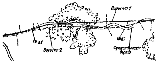
Рис. 2.1. Варианты исправления трассы в плане.
