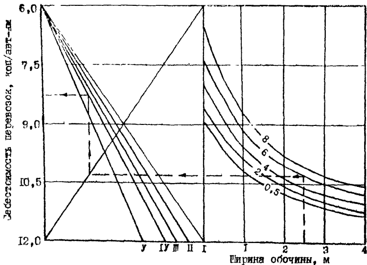
Рис.9.8. Номограмма для определения себестоимости перевозок при различном состоянии обочины /цифры на кривых - интенсивность движения в тыс.авт/сутки/: I - обочины укреплены, имеются краевые полосы, покрытие такое же, как на проезжей части; II - обочины укреплены щебнем, краевые полосы отсутствуют; III - обочины засеяны травой; IV - неукрепленные сухие обочины; V - неукрепленные влажные обочины.
