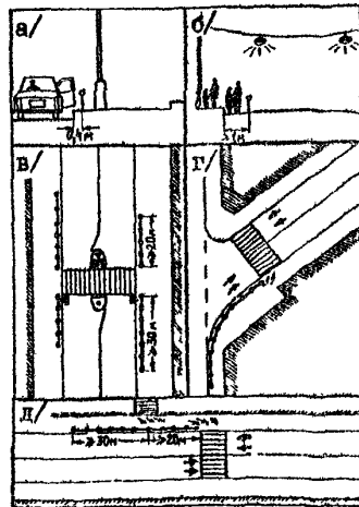
Рис.8.2. Схемы установки ограждений у пешеходных переходов.
