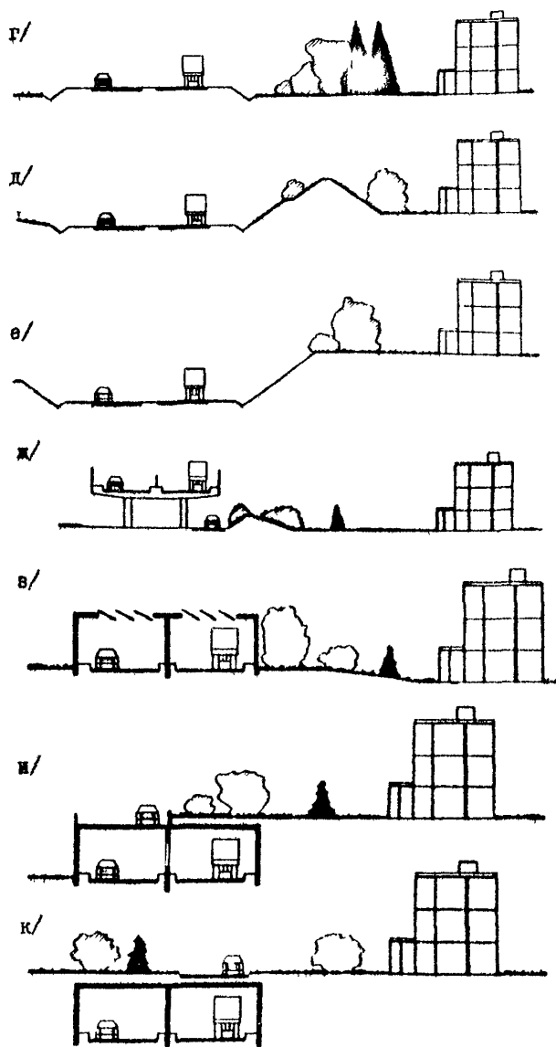
Рис. б,2. Принципиальные схемы защиты застройки от транспортного шума.
