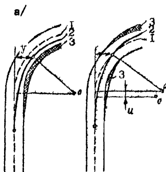
Рис.2.10. Особенности расположения переходной кривой при реконструкции дорог: а - обычный способ вписывания переходной кривой; б - вписывание переходной кривой со смещением центра круговой кривой; 1 - исходная ось полосы движения; 2 - ось полосы движения после введения переходной кривой; 3 - улитрава покрытия.
