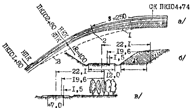
Рис.2.11. Оформление проекта устройства срезки видимости: а - план кривой; б - срезка откоса выемки на ПК 104+74 для обеспечения видимости; в - вырубка деревьев для обеспечения видимости; 1 - граничная кривая видимости; 2 - начало ограничения видимости откосами выемки; 3 - граница вырубki леса для обеспечения видимости; 4 - срезка откосов; 5 - ось дороги; 6 - уширение проезжей части; 7 - траектория движения автомобиля.
