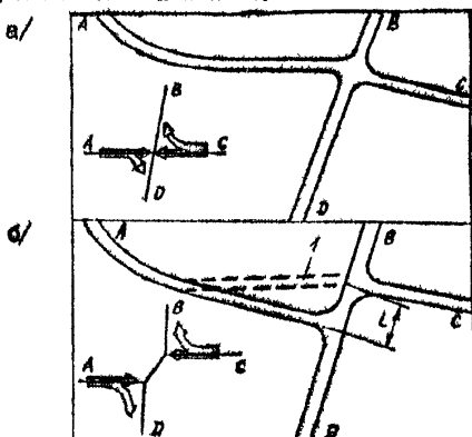
Рис.2.14. Перестройка пересечения на два смещенные примыкания: а - первоначальная планировка; б - планировка после реконструкции; I - закрытый участок дороги; в левых нижних углах показаны стрелы грузопотоков.
