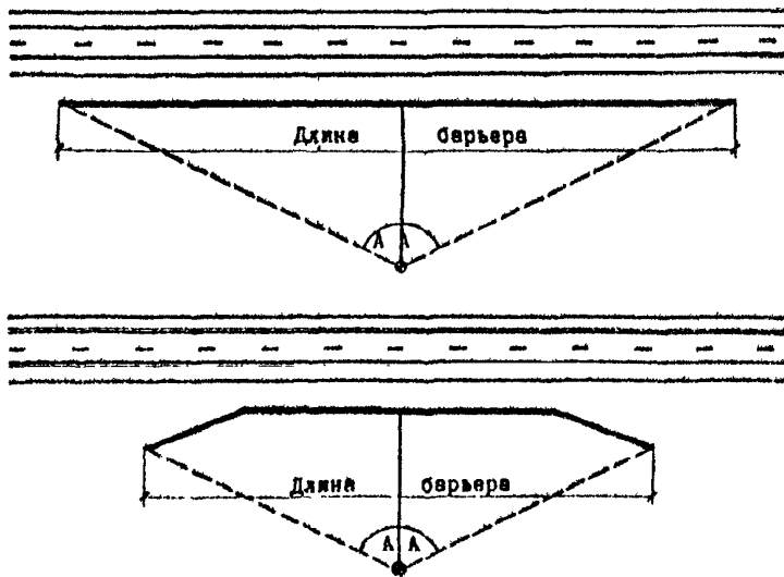
Рис.10.7. График для определения снижения уровня звука препятствием ограниченной длины
