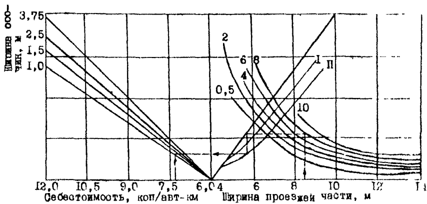
Рис.9.1. Номограмма для определения себестоимости перевозок при различной ширине проезжей части и обочины/ширины на кривых - интенсивность движения в тыс.авт/сутки/: I - краевые полосы по 0,8 м; II - краевые полосы по 0,5
