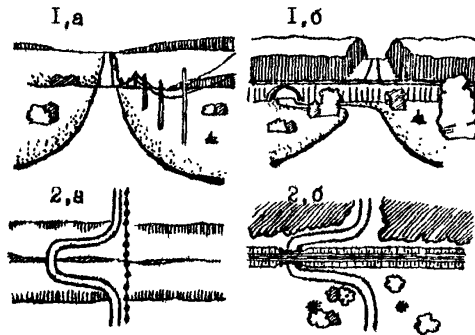
Рис. 2.4. Неправильное представление у водителей о направлении дороги, вызванное скрытым поворотом дороги: а - невидимый водителю издалека поворот; б - невидимый ночью поворот дороги под железнодорожный мост; 1 - вид дороги; 2 - план дороги.
