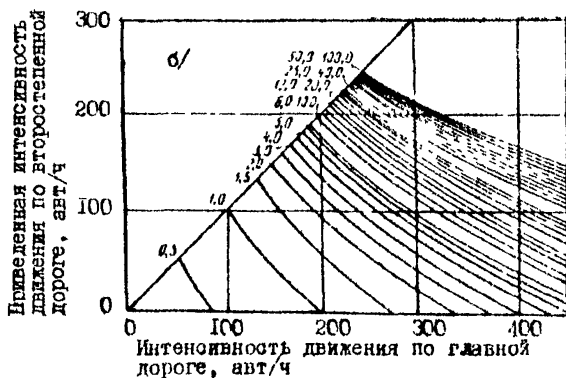
Рис.9.8. Графики для определения потерь времени на пересечениях в одном уровне (цифры на кривых - потери времени в авт-ч); а - неоснащенные пересечения; б - частично и полностью канализированные пересечения.
