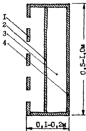
Рис. 5.4. Конструкция элемента шумопоглощающего барьера: 1 - внешняя фронтальная рама; 2 - внутренний поглощающий материал; 3 - слой воздуха; 4 - задняя внешняя рама.
