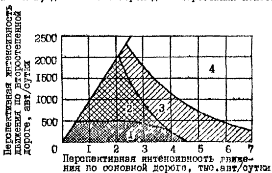
Рис.2.18. Области применимости различных планировочных решений пересечений в одном уровне: 1 - простые пересечения; 2 - пересечения с направляющими островками; на второстепенной дороге; 3 - пересечения с направляющими островками на обеих дорогах, переходно-скоростными полосами и дорожной разметкой; пересечения со светофорным регулированием или в разных уровнях
