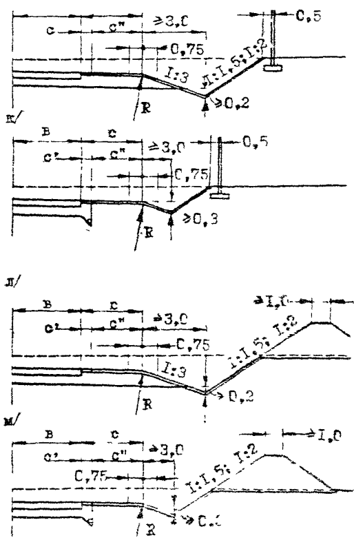
Рис. 5.7. Реконструкция поперечного профиля земляного полотна: а, б, в, г, д, е, з - насыпь высотой до 2 м; и, к, л, м, н - выемки глубиной до 1 м; п - сочетание грунтового вала с шпуровальными сарьяром.
