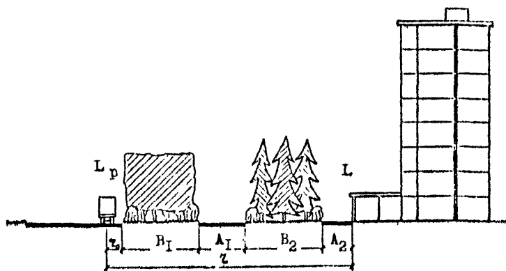
Рис.10.1. Расчетная схема к определению эффективности зеленых насаждений.
