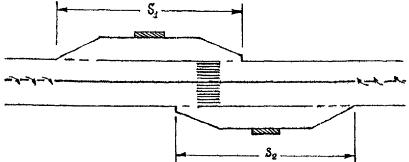
Рис. 3.3. Планировка автобусных остановок и разметка проезжей части в их зоне.
