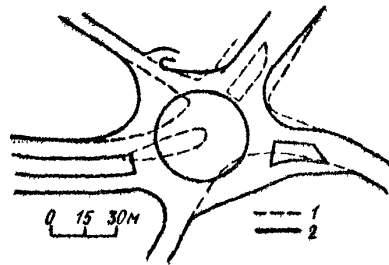
Рис.2.19. Реконструкция пересечения нескольких дорог в пересечение кольцевого типа: 1 - планировка пересечения до реконструкции; 2 - планировка после реконструкции.
