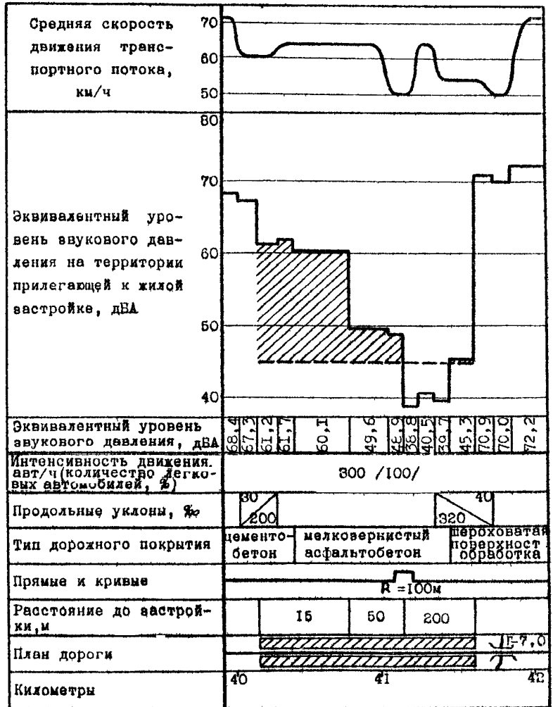
Рис.Б.1. Линейный график изменения эквивалентного уровня звука в районе жилой застройки вдоль дороги
