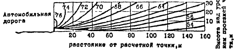
Рис.10.3. Распространение шума от транспорта при интенсивности движения 3000 авт/ч: а - без шумозащитного барьера; б - с шумозащитным барьером высотой 4 м
