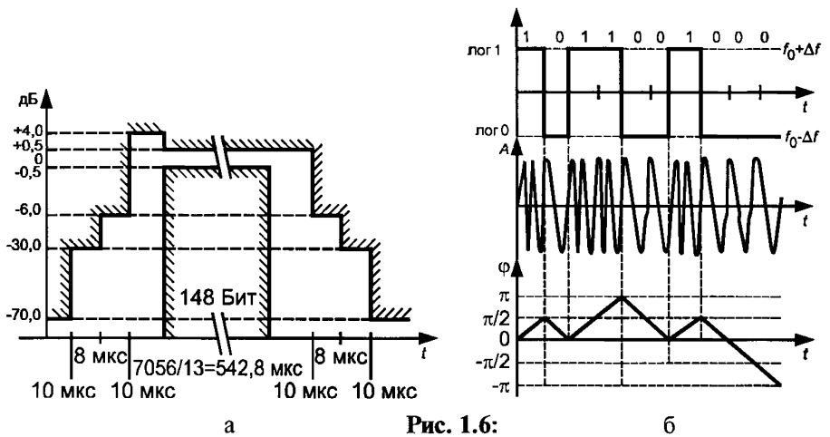
Рис. 1.6: а — маска огибающей радиочастотного пакета; б — информационная часть радиочастотного пакета
