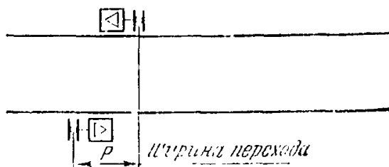
Рис. 8.11. Размещение знаков 5.16.1 и 5.16.2 на неразмеченном пешеходном переходе
