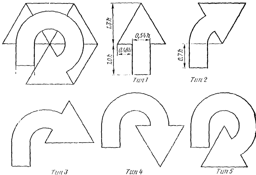
Рис. 19.1. Принцип построения стрелок для знаков 5.20.2 и 5.21.2
