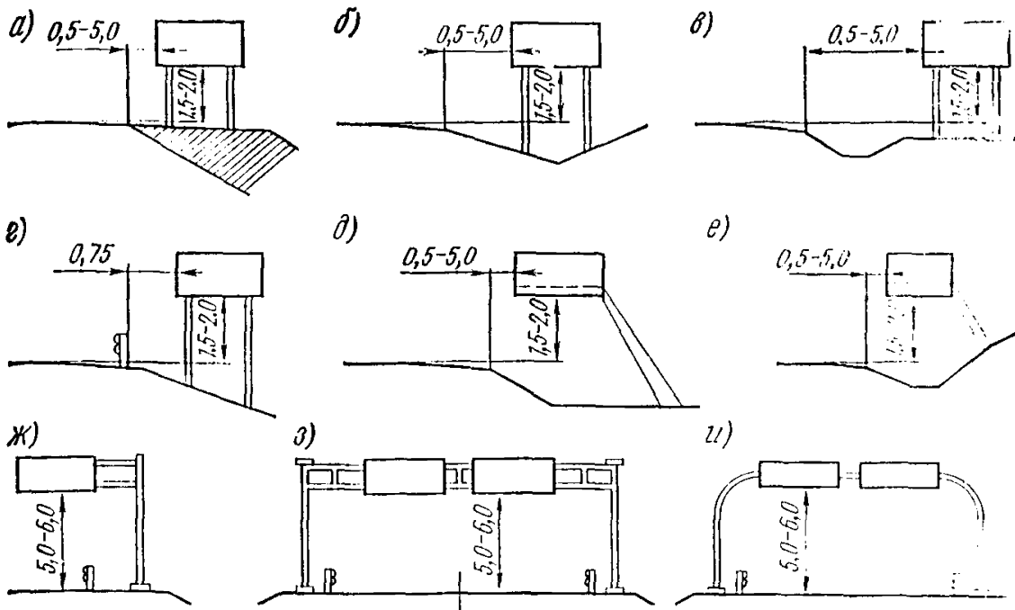
Рис. 3.4. Способы установки предварительных указателей направлений
