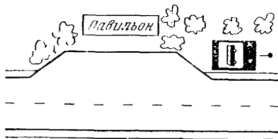
Рис. 8.10. Размещение знака 5.12 у начала остановочной площадки
