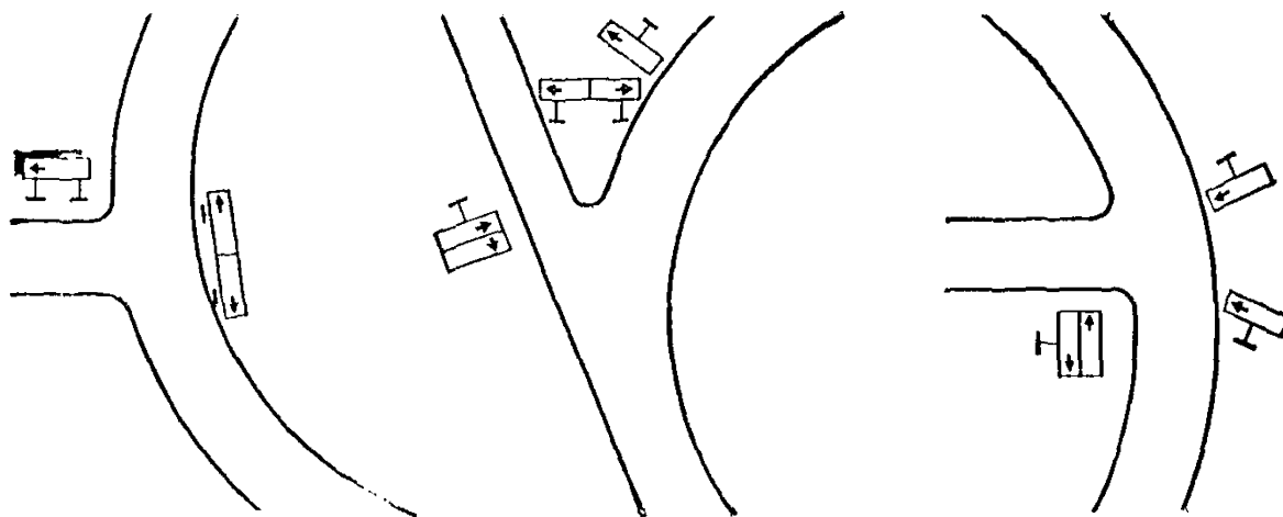
Рис. 13.6. Схемы установки знаков 5.21 «Указатель направлений» на примыканиях двух-, трехполосных дорог
