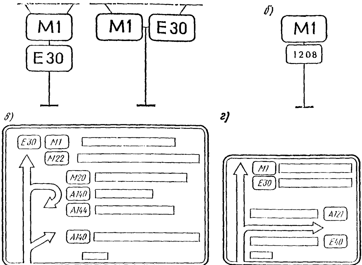
Рис. 19.10. Примеры расположения знаков 5.29.1:
