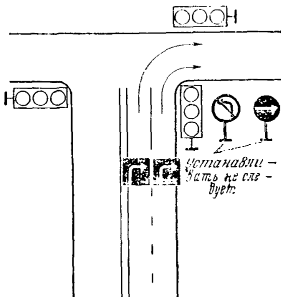
Рис. 8.7. Применение знака 5.8.1 в ситуации, когда установка знака 3.18.2 или 4.1.2 делала возможным поворот только из правой полосы
