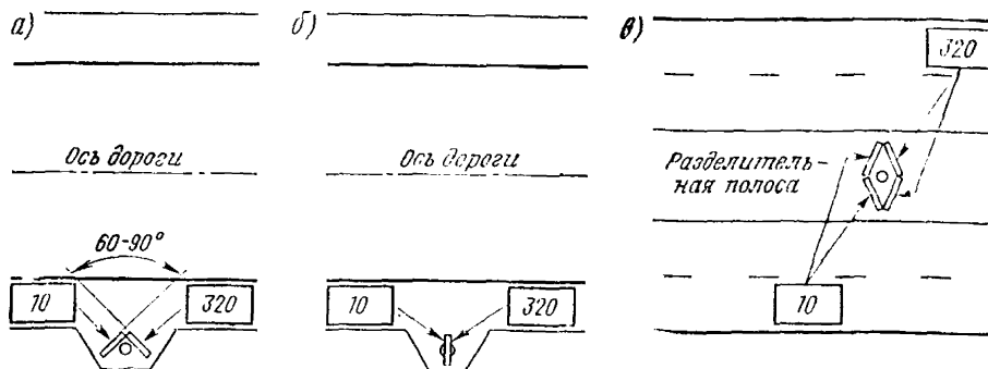
Рис. 8.13. Способы установки километровых знаков на автомобильных дорогах
