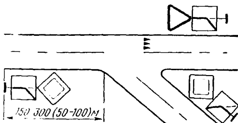
Рис. 5.1. Установка знаков приоритета в местах изменения направления главной дороги
