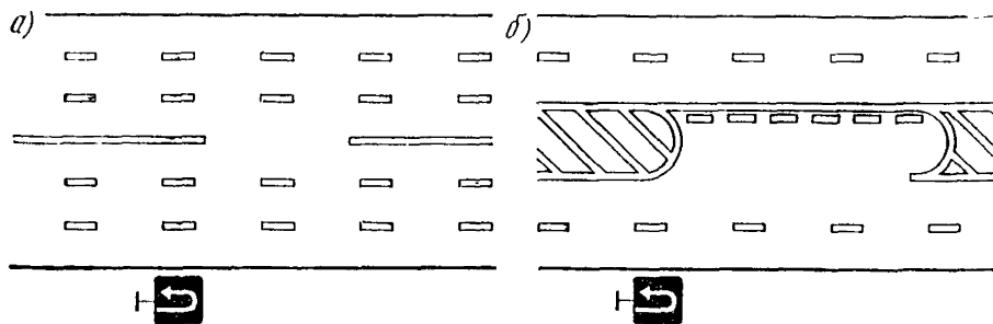
Рис. 8.9. Схемы установки знака 5.11 «Место разворота»
