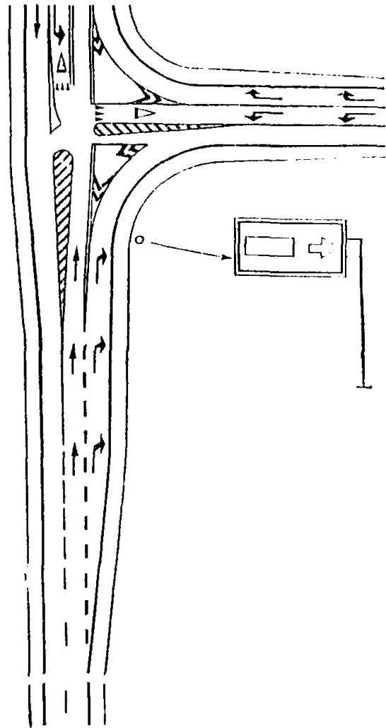
Рис. 13.4. Размещение знака 5.21.2 на Г-образной опоре
