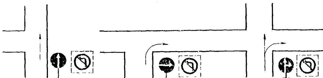
Рис. 7.1. Применение знаков 4.1.1, 4.1.2 и 4.1.4 для запрещения поворота налево и разворота (знак 3.18.2 не устанавливается)
