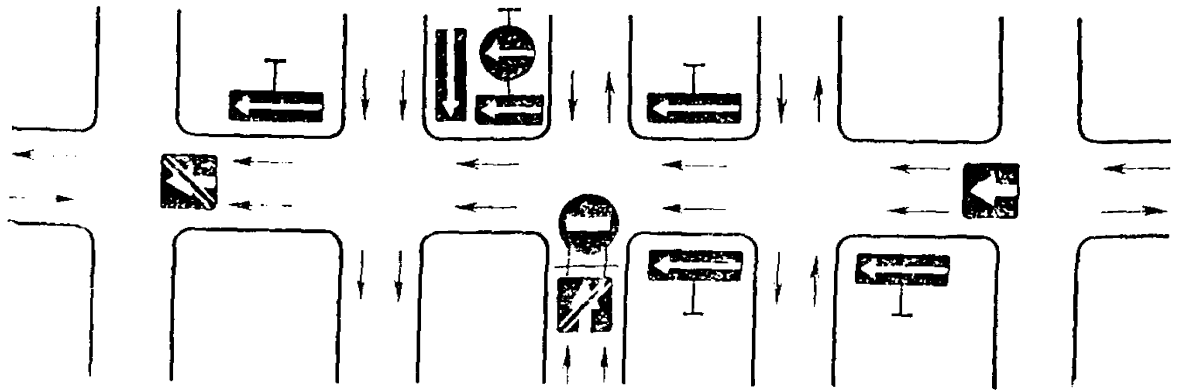
Рис. 8.3. Пример организации одностороннего движения
