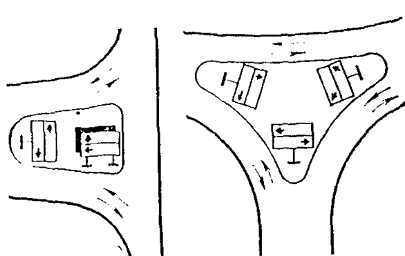
Рис. 13.7. Схемы установки знаков 5.21 «Указатель направлений» на примыканиях с островками безопасности
