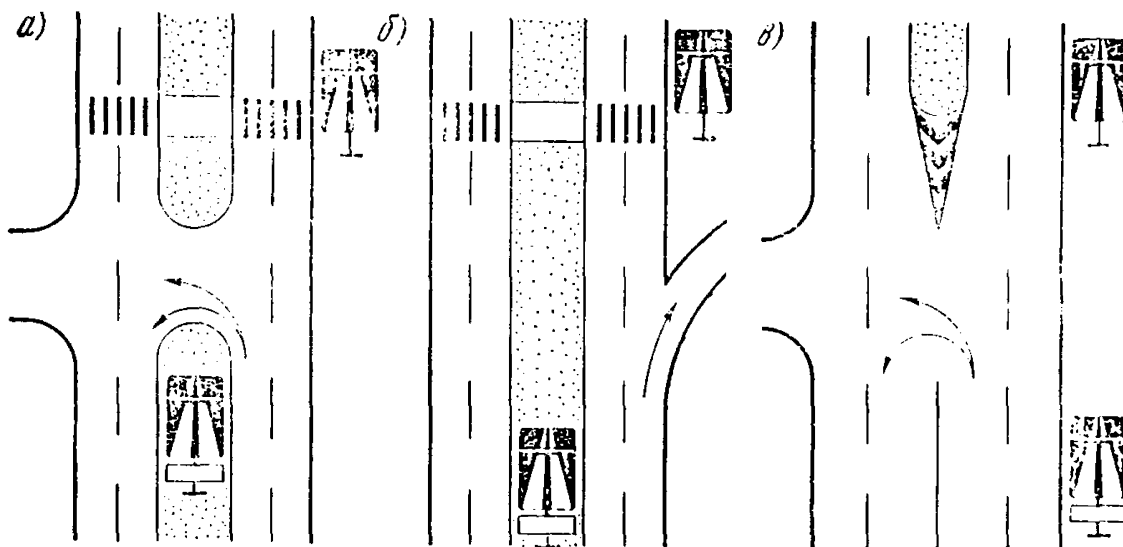
Рис. 8.1. Схемы установки знака 5.1 «Автомобильная дорога»
