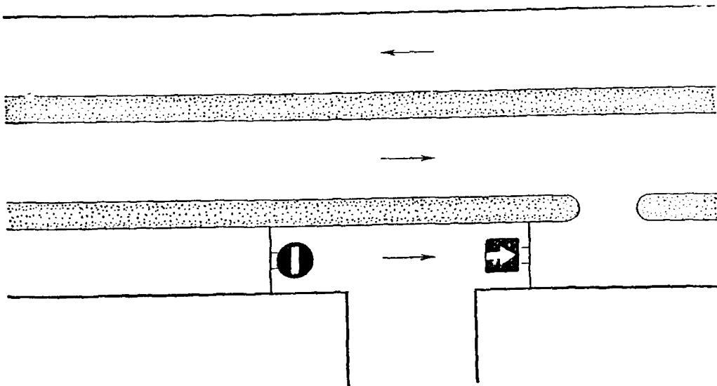
Рис. 6.3. Установка знака 3.1 при организации одностороннего движения по боковому проезду на дороге с несколькими проезжими частями
