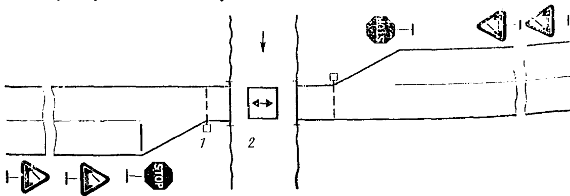
Рис. 17.1. Схема установки знаков на паромной переправе:
