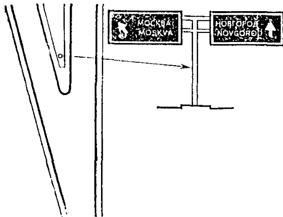
Рис. 13.5. Размещение знаков 5.21.2 на Т-образной опоре
