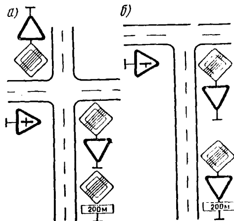
Рис. 13.9. Установка знаков приоритета в месте пересечения дорог, ранее объявленных главными с помощью знака 2.1:
