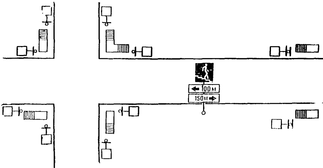
Рис. 8.12. Пример применения знаков 5.17.1 и 5.17.2
