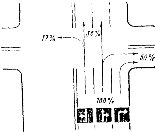
Рис. 8.4. Распределение полос по направлениям движения в зависимости от интенсивности движения
