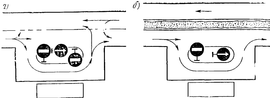
Рис. 6.4. Использование знака 3.1 для организации одностороннего въезда и выезда с площадки: а — на дорогах без разделительной полосы; б — на дорогах с разделительной полосой
