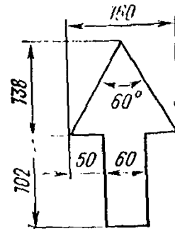
Рис. 19.9. Размеры стрелки для знака 5.29.2
