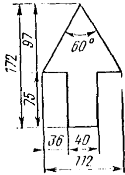
Рис. 19.8. Размеры стрелки для знаков 5.21.2, применяемых в городской подсистеме ориентирования
