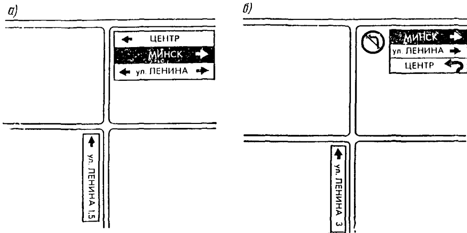
Рис. 12.10. Знаки 5.21.2 с указанием направления к вылетной магистрали, название которой не связано с названием конечного пункта:
