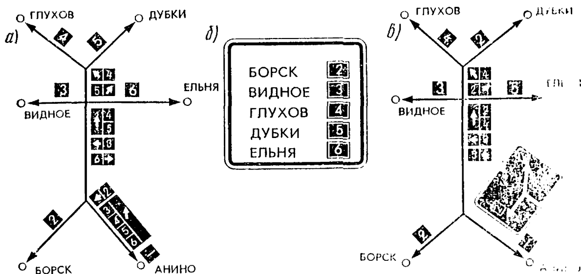
Рис. 12.7. Схема нумерации маршрутов в населенном пункте и оборудования их знаками. Указаны знаки, предназначенные только для водителей, которые въезжают в населенный пункт с направления Анино:
