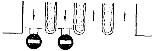
Рис. 6.2. Установка знаков 3.1 при наличии нескольких проезжих частей с односторонним движением
