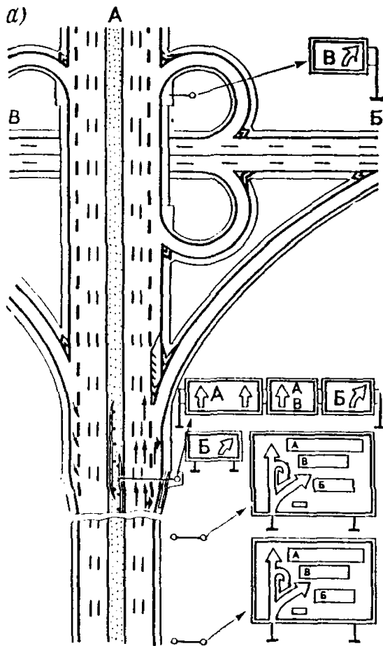
Рис. 14.1. Примеры применения указателей направлений:
