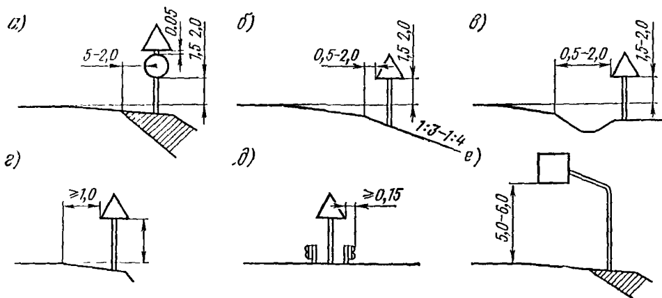
Рис. 3.3. Способы установки знаков на дорогах вне населенных пунктов
