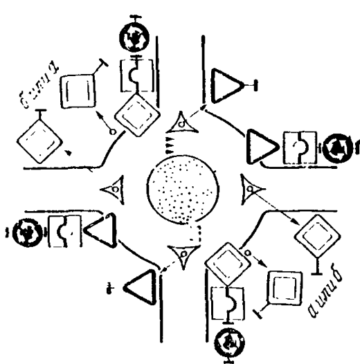
Рис. 13.12. Установка знаков на кольцевом пересечении при прохождении главной дороги в прямом направлении:
