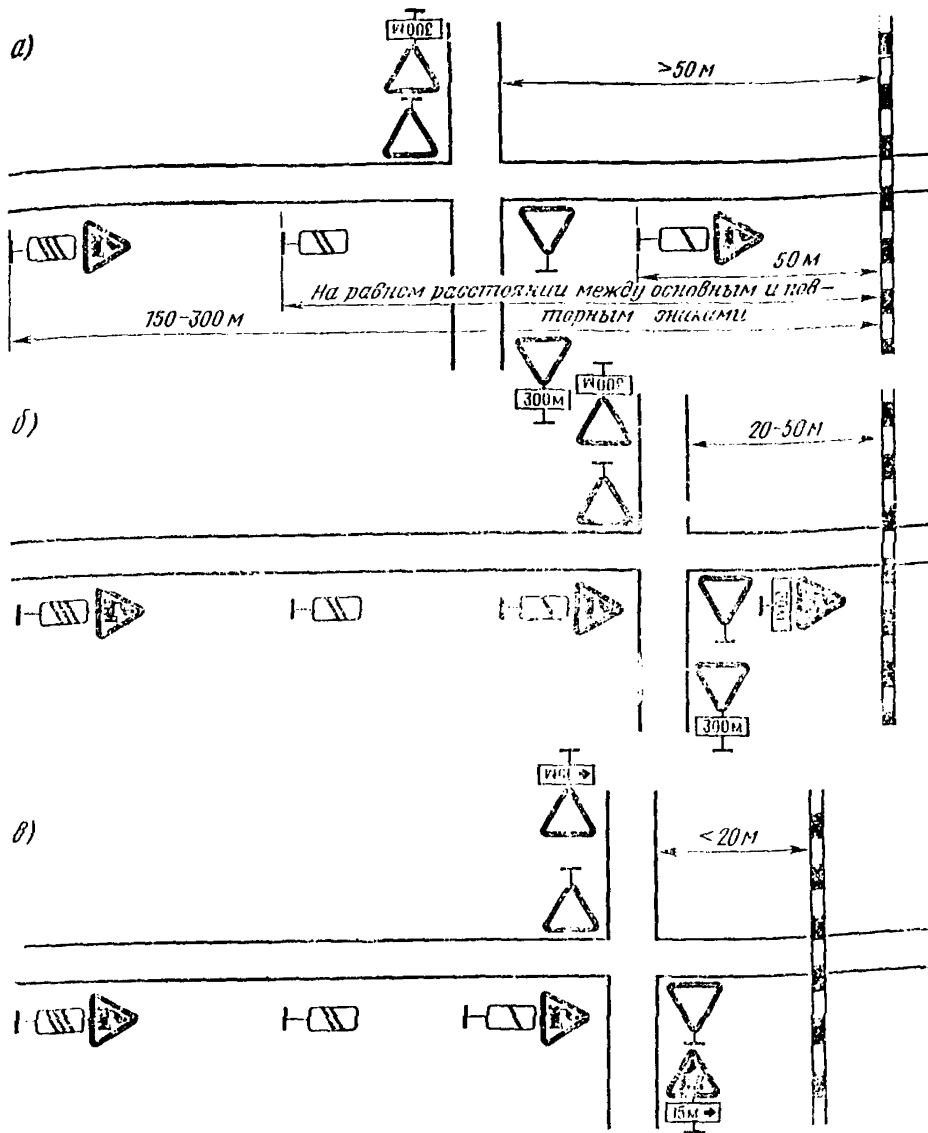
Рис. 16.1. Расположение знака 1.1 или 1.2 при прохождении автомобильной дороги параллельно железной:
