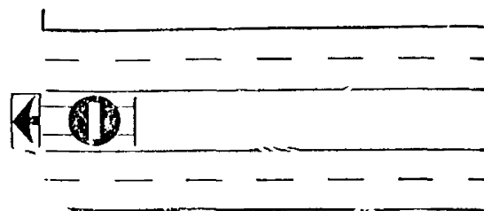
Рис. 6.4. Использование знака 3.1 для организации одностороннего въезда и выезда с площадки: а — на дорогах без разделительной полосы; б — на дорогах с разделительной полосой
