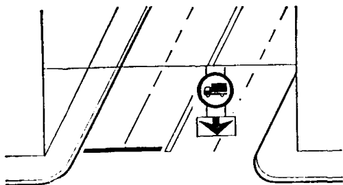
Рис. 6.8. Установка знака 3.4 с табличкой 7.14 для запрещения движения грузовых автомобилей по отдельной полосе проезжей части
