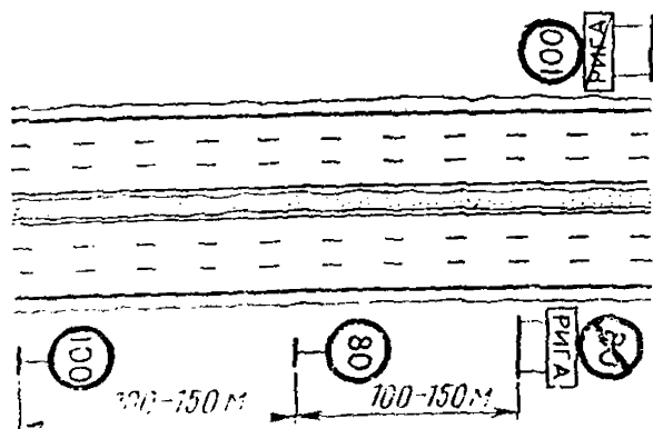
Рис. 6.13. Установка знаков в конце участка с повышенным скоростным режимом
