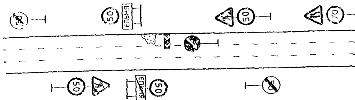
Рис. 6.14. Подтверждение пониженного предела скорости в начале населенного пункта
