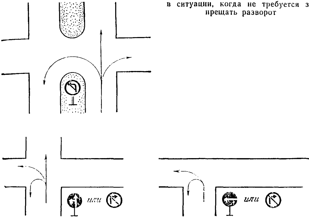
Рис. 7.3. Ситуации, в которых предпочтение следует отдавать предписывающим знакам
