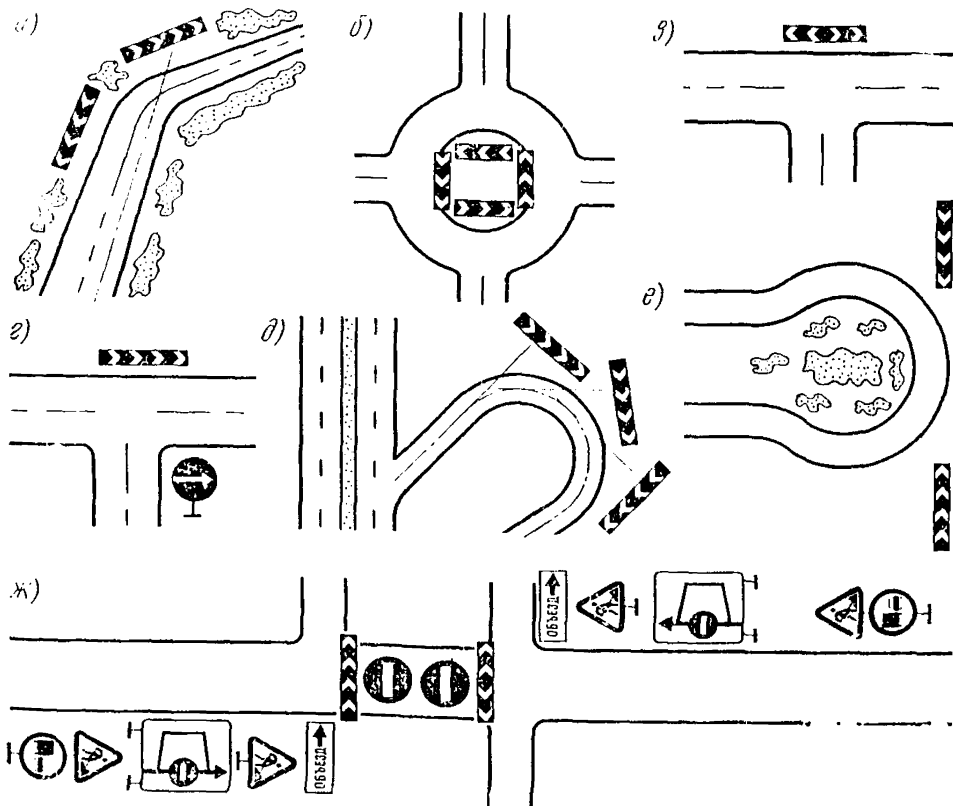
Рис. 4.1. Примеры применения знаков 1.31.1—1.31.3:
