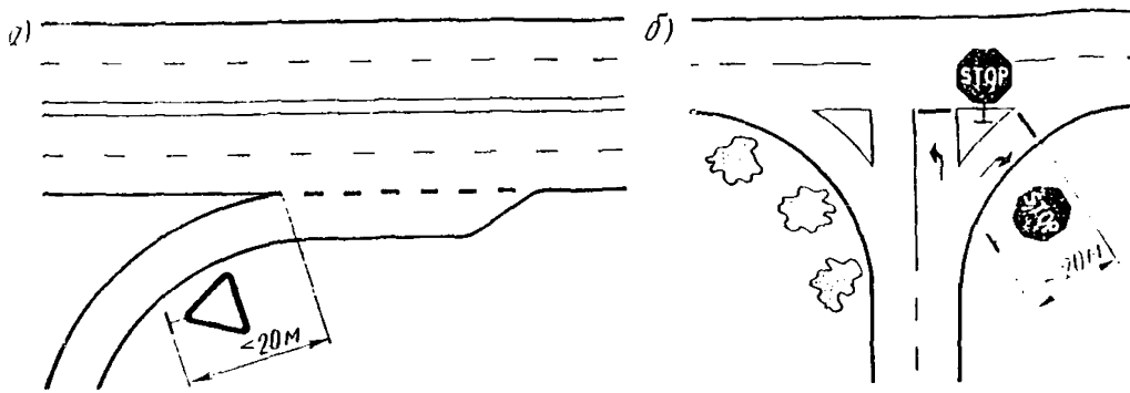
Рис. 5.2. Установка знаков 2.4 и 2.5 при выезде на пересекаемую дорогу под острым углом:
