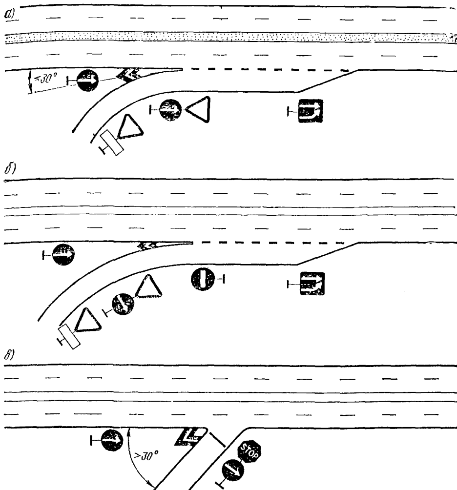
Рис. 14.2. Примеры применения знаков на примыканиях соединительных съездов:
