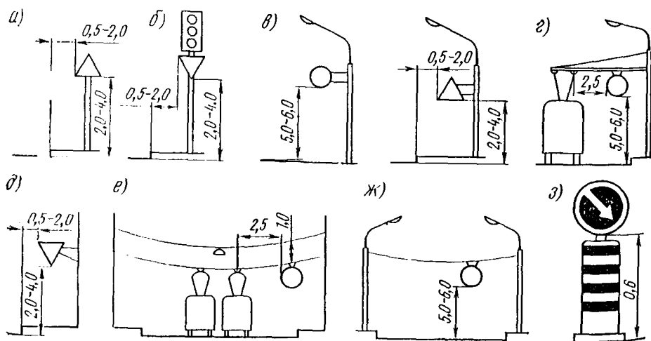
Рис. 3.6. Способы установки знаков в населенных пунктах
