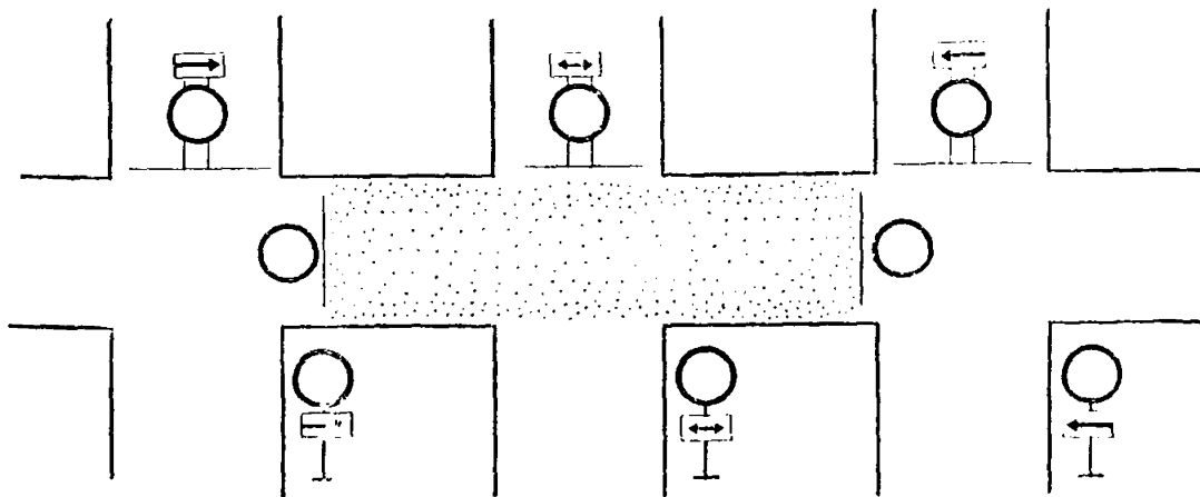
Рис. 6.7. Установка знаков 3.2 со всех направлений при закрытии участка дороги для движения транспортных средств
