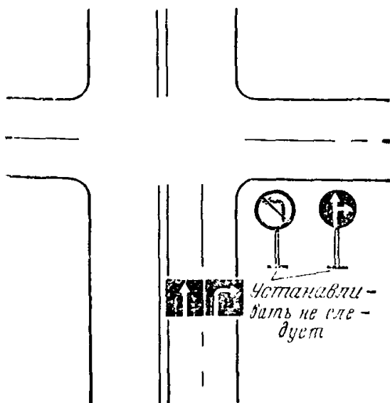
Рис. 8.6. Пример применения знаков 5.8.1 или 5.8.2, установка знаков 3.18 или 4.1 при этом исключается
