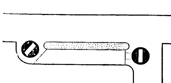
Рис. 6.5. Установка знаков 3.1 на развортно-отстойных площадках, предназначенных для транспортных средств общего пользования, движущихся по установленным маршрутам
