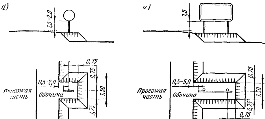
Рис. 3.5. Устройство берм для установки знаков:
