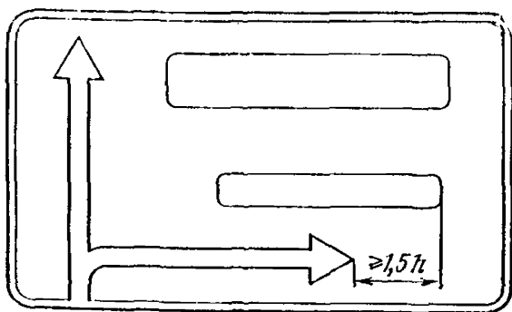
Рис. 19.6. Пример компоновки знака 5.20.1
