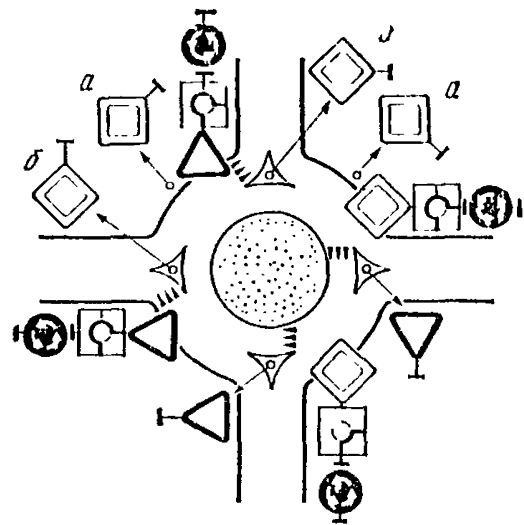
Рис. 13.13. Установка знаков на кольцевом пересечении в случае, когда главная дорога изменяет свое направление:
