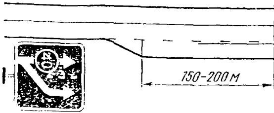
Рис. 8.8. Организация движения на подъеме с помощью знака 5.8.3
