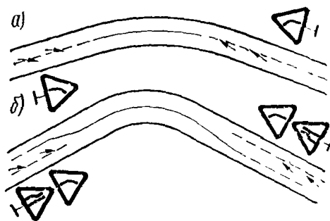
Рис. 15.1. Схемы установки знаков на горизонтальных кривых:
