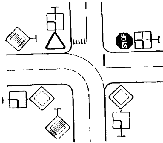
Рис. 13.10. Установка знаков приоритета на отдельном перекрестке при изменении направления главной дороги
