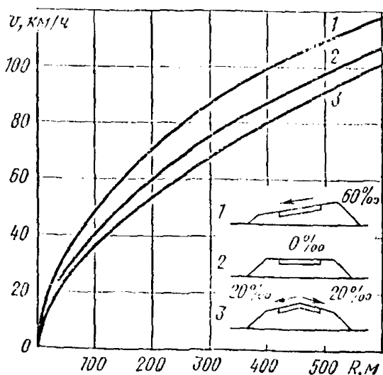
Рис. 6.11. Выбор верхнего предела скорости движения на кривых
