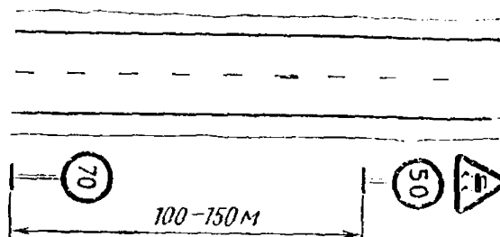
Рис. 6.12. Ступенчатое ограничение скорости
