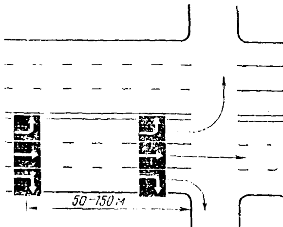
Рис. 8.5. Расположение знаков 5.8.2 относительно перекрестка
