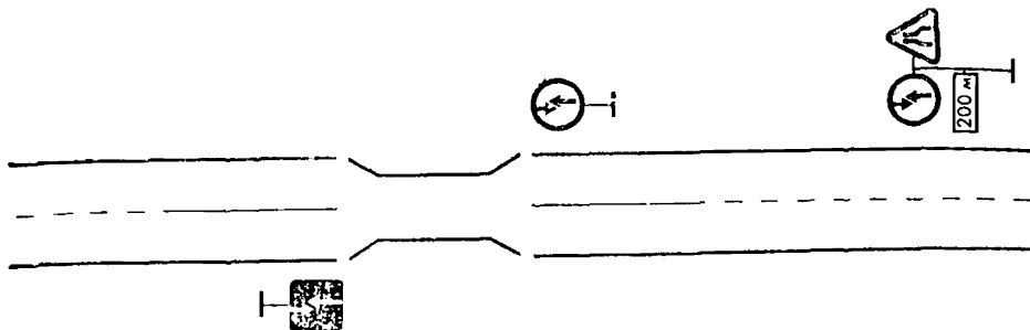
Рис. 5.3. Пример предварительной установки знака 2.6
