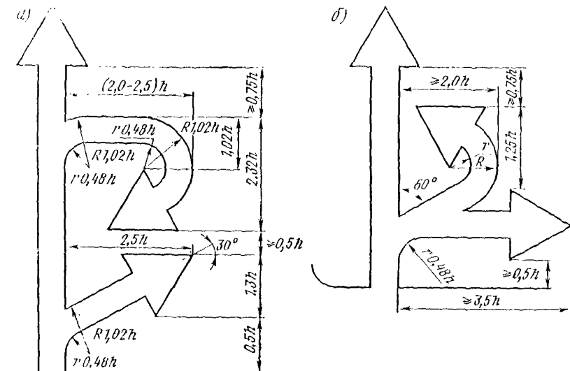
Рис. 19.2. Рекомендуемая конфигурация стрелок на знаке 5.20.1, устанавливаемом перед развязкой в разных уровнях, с точки зрения сокращения размеров знака и улучшения его информативности (возможно горизонтальное расположение нижней стрелки в варианте а)
