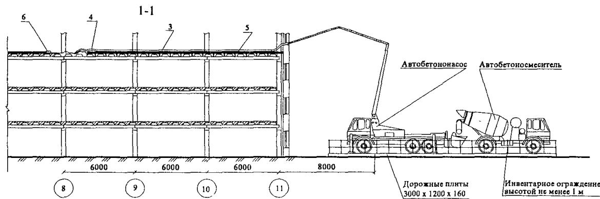
Рисунок 5 – Производство работ по бетонированию плиты перекрытия
