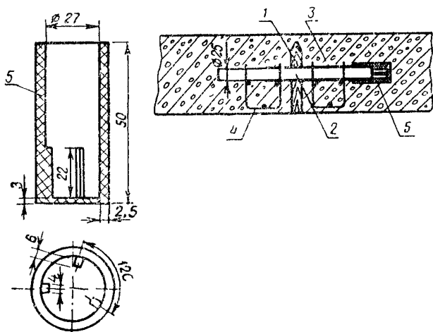
Рис. 9. Схема установки стального стержня с резиновым колпачком в цементобетонное покрытие.
