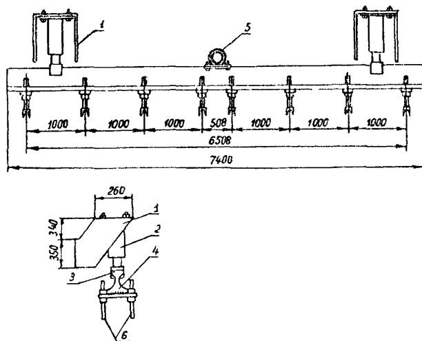
Рис. 10. Схема приспособления для погружения штырей (конструкция СУ-818 треста «Югозапдорстрой» Главдорстроя):
