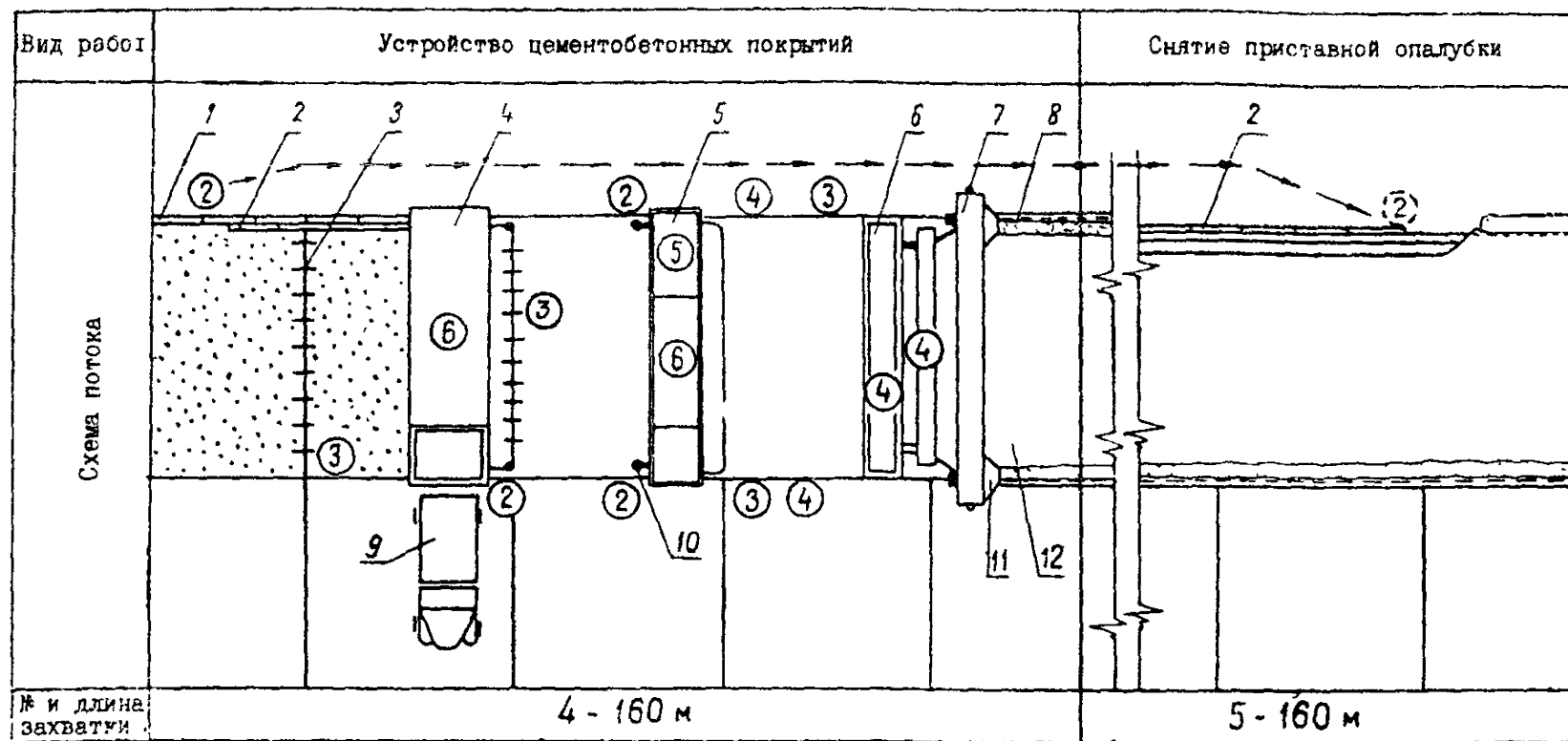
Рис. 8. Технологическая схема устройства цементобетонного покрытия:
