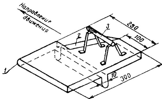
Рис. 11. Мастерок для отделки продольного шва 1—закругляющая кромка для заглаживания свежего бетона; 2—заточенная кромка для очистки поверхности затвердевшего бетона; 3—ручка, смещенная на затвердевшую плиту
