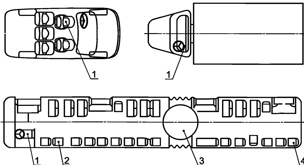
1 — точка отбора проб для АТС категорий М, N; 1,2,4 — точки отбора проб для АТС категорий М 2 , М 3 ; 3 — точка отбора проб для АТС категории М 3 (сочлененный)
