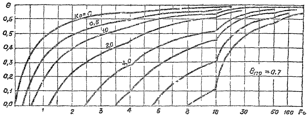
Рис. 10 Нестационарные температурные поля под центрами источников в форме полосы, прямоугольника, круга, их заглубленных аналогов, а также - горизонтальных труб в грунте при \partial_{\tau p} = 0,7 и \partial_{\tau r} = 0,4 .
