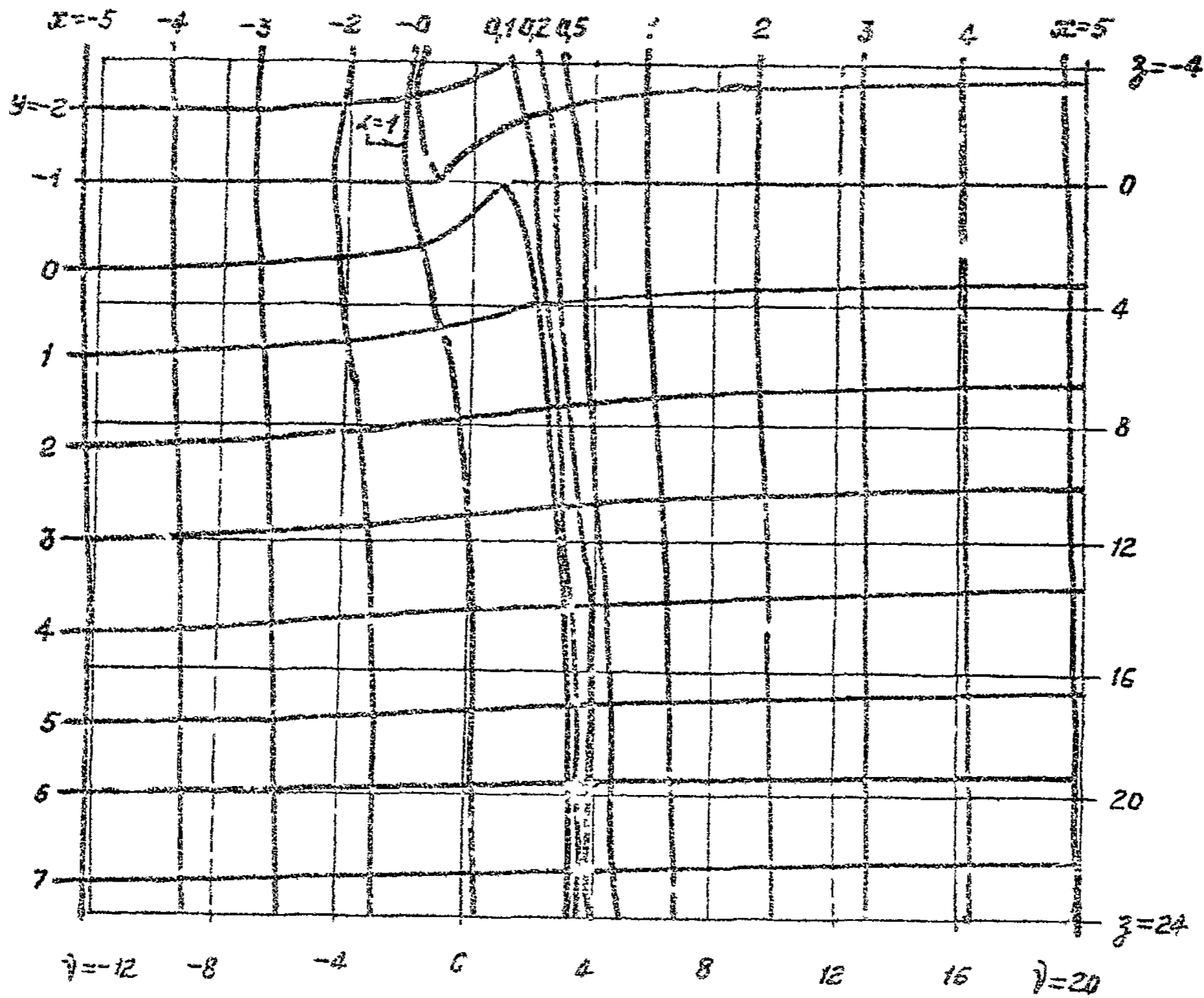
Рис.3 Сетка для перевода координат X, Y в координаты z, v и обратно.
