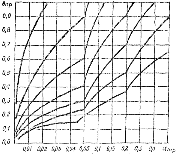
Рис. 2 Стационарные (предельные) температурные поля под центром ( x=0 ) горизонтальной трубы в области y \geq z_{тр} \cdot h_{тр}, a_{тр} \frac{h_{тр}^2 - z_{тр}^2}{y^2}
