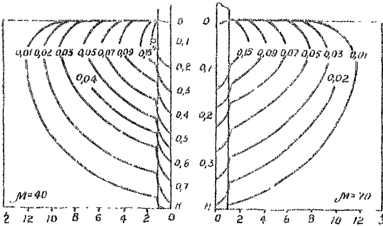
Рис.6 Стационарные (предельные) температурные поля в системе грунт-термосыя при t_{\text{вн}} = 22
