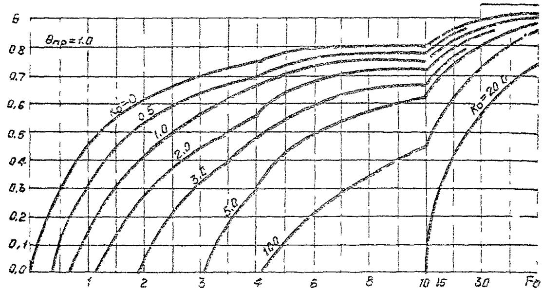
Рис.7 Нестационарные температурные поля под центрами источников в горючей полосе, прямоугольника, круга, их заглубленных аналогов и также горизонтальной трубы в грунте при \theta_{0p} = 1 и \theta_{0p} = 0,1 .
