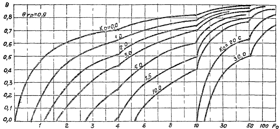
Рис. 8 Нестационарные температурные поля под центрами источников в форме полосы прямоугольника круга, их заделанных аналогов, а также горизонтальной трубы в трубе при Bi_p = 0,9 и Bi_p = 0,2
