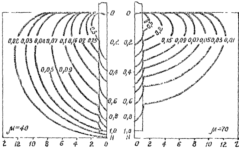
Рис.4 Стационарные (предельные) температурные поля в системе грунт-термосвая при \frac{q}{j} = 8
