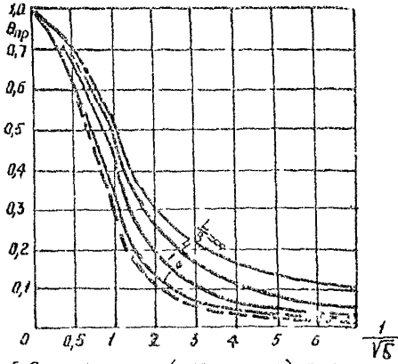
Рис. 1 Стационарные (предельные) температурные поля под центрами ( x = 0,5b, z = 0 ) поверхностных источников.
