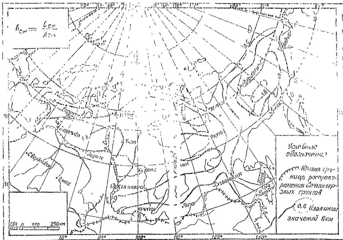
Рис.18 Изолинии значения K_{CH} на территории с вечной мерзлыми грунтами
