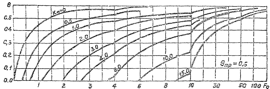
Рис. II Нестационарные температурные поля под центрами источников в форме полусп. прямоугольника, круга, их закругленных аналогов а также - горизонтальной трубы в грунте при \theta_{пр} = 0.5 = \theta_{гд} = 0.5
