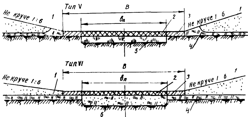
Рис.2. Поперечные профили автозимников, прокладываемых по заболоченным поймам и долинам рек: 1-снеговой покров; 2-тщательно укатанный снег на проезжей части; 3-уплотненный снег на обочинах; 4-естественный мохорастительный покров; 5-лед; 6-перемешанный с мохорастительным покровом грунт, тщательно спланированный гладилками
