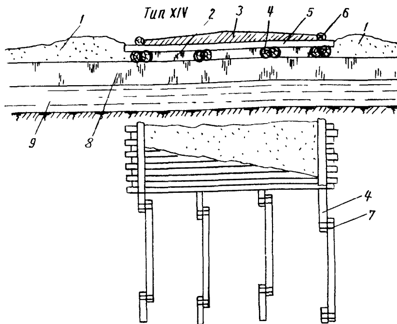
Рис.8. Конструкция "плавающей" дерево-ледяной переправы: 1-валик из снега; 2-намороженный слой льда; 3-грунтовая за- сыпка; 4-продольные лежни: d = 20-22 см; 5-сплошной сланевый настил из тонкомерной древесины d = 12-16 см; 6-колесоотбой- ные брусья d = 22-24 см; 7-проволочная скрутка d = 8 мм; 8-ес- тественный ледяной покров; 9-вода
