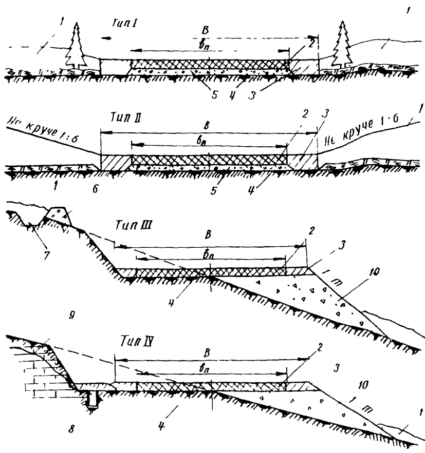
Рис.1. Поперечные профили автозимняков на прочных грунтовых основаниях:
