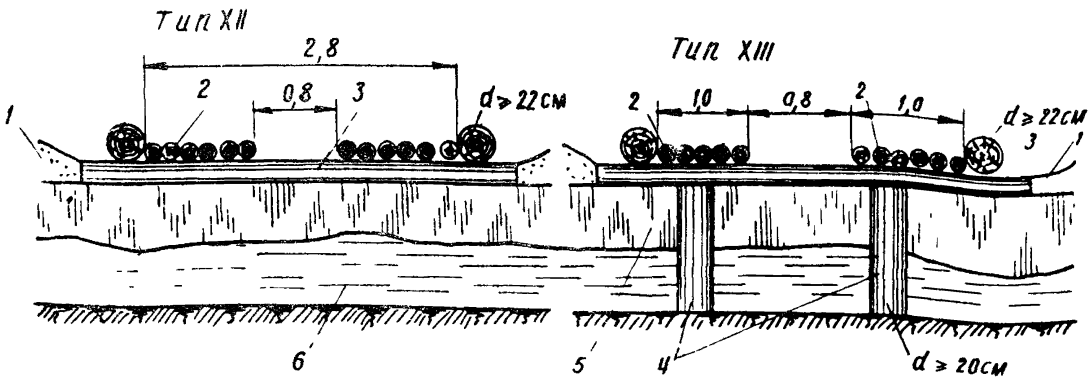
Рис.7. Поперечные профили автозимников на ледяном покрове (ледяные переправы) при устройстве деревянного настила:
