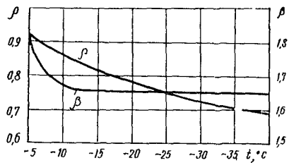
Рис.13. График для определения коэффициентов \rho и \beta
