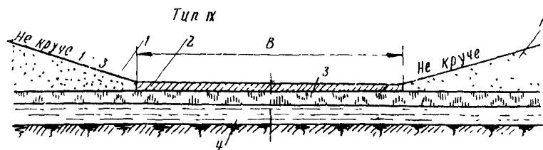
Рис.5. Поперечный профиль автозимника на ледяном покрове рек и озер: 1-снеговой покров; 2-уплотненный слой снега на полотне; 3-ледяной покров; 4-вода
