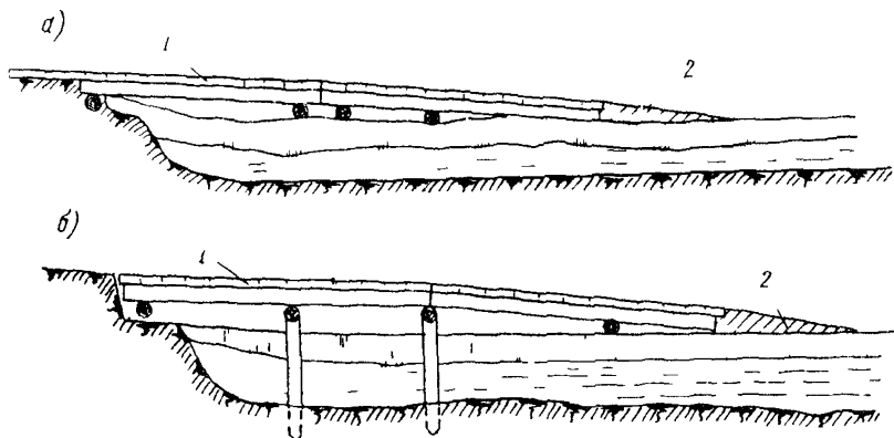
Рис.9. Конструкции сопряжения берега и ледяного покрова на переправах:
