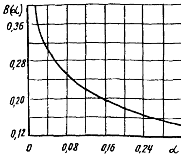
Рис.11. График для определения коэффициента B(\alpha)
