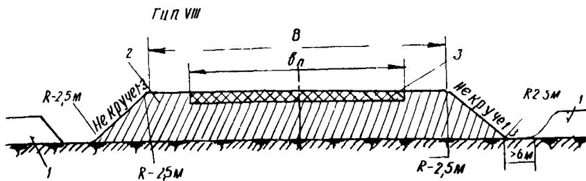
Рис.4. Поперечный профиль автозимника в насыпи из снега 1-снеговой покров; 2-насыпь из уплотненного снега; 3-оледененный слой снега на проезжей части или настил из тонкомерной древесины, веток, сучьев и т.п.
