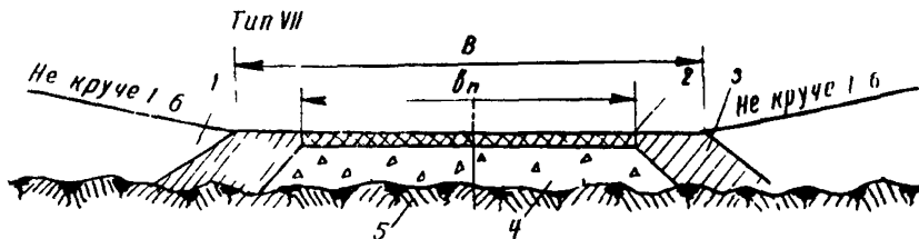
Рис.3. Поперечный профиль автозимника на марях и бугристых вечномерзлых торфяниках:
