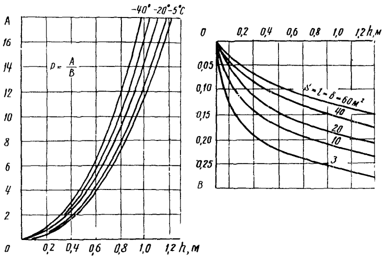
Рис.12. Графики для определения параметров A и B
