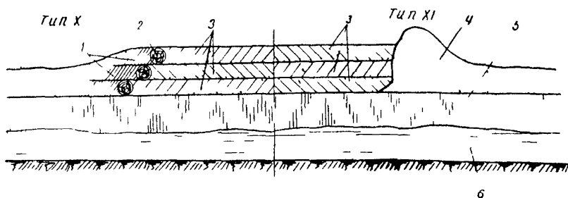
Рис.6. Поперечные профили автозимников на ледяном покрове (ледяные переправы) при усилении методом послойного намораживания льда.
