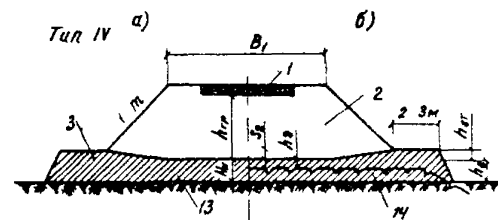
Рис.1. Поперечные профили дорог на промороженных основаниях: а—состояние конструкции на конец холодного периода года, б—то же, на конец теплого периода 1—дорожная одежда, 2—минеральная часть земляного полотна, 3—намороженная торфяная плита, 4—промороженный слой торфяной залежи, 5—талый слой торфяной залежи, 6—боковые теплоизолирующие призмы из торфа, 7—боковой резерв (водоотводная канава), 8—талая торфяная прослойка за счет оттаивания сверху; 9—то же, за счет оттаивания снизу; 10—минеральное дно болота; 11—выдавливаемые торфяные отложения или вода; 12—послойно намороженная плита из торфа устойчивой консистенции взамен жидких образований, 13—поверхность вечномерзлых торфяников, 14—верхняя граница мерзлых грунтов после постройки дороги
