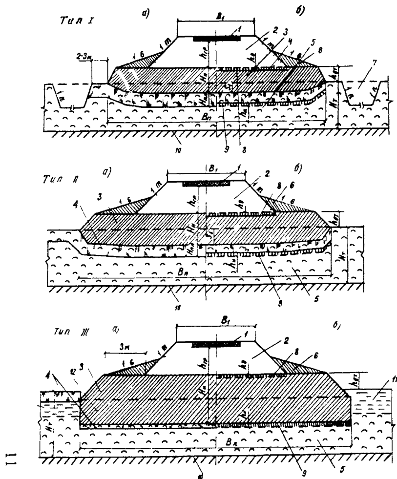
Рис.1. Поперечные профили дорог на промороженных основаниях: а—состояние конструкции на конец холодного периода года, б—то же, на конец теплого периода 1—дорожная одежда, 2—минеральная часть земляного полотна, 3—намороженная торфяная плита, 4—промороженный слой торфяной залежи, 5—талый слой торфяной залежи, 6—боковые теплоизолирующие призмы из торфа, 7—боковой резерв (водоотводная канава), 8—талая торфяная прослойка за счет оттаивания сверху; 9—то же, за счет оттаивания снизу; 10—минеральное дно болота; 11—выдавливаемые торфяные отложения или вода; 12—послойно намороженная плита из торфа устойчивой консистенции взамен жидких образований, 13—поверхность вечномерзлых торфяников, 14—верхняя граница мерзлых грунтов после постройки дороги
