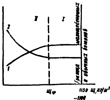
Рис.1. Зависимость подвижности OK (осадки конуса) (1) и жесткости Ж (2) бетонной смеси от содержания щебня \Delta C :
