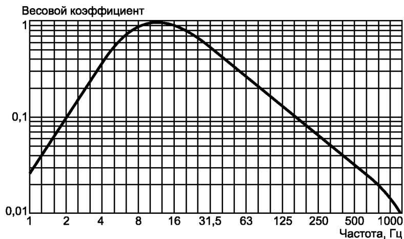
Рисунок В.2 — Функция частотной коррекции W_h для определения параметров локальной вибрации
