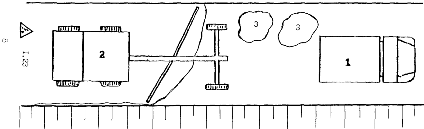
1 - автомобиль самосвал; 2 - автогрейдер ДЗ-61А; 3 - грунт.
