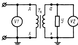
V1, V2 —образцовые вольтметры.
