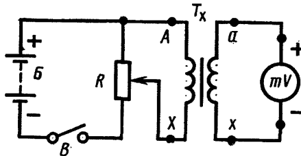
Б —источник питания постоянного тока; В —выключатель; R —регулируемый резистор; Т х —поверяемый трансформатор напряжения; mV —милливольтметр.
