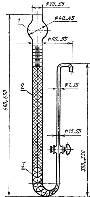
1 — анализируемый раствор; 2 — катионитовая смола; 3 — стеклянная вата
