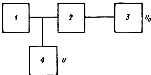
1—источник напряжений; 2—образцовый делитель напряжения; 3—образцовый вольтметр для измерения малых напряжений; 4—поверяемый вольтметр
