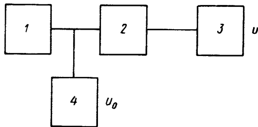
1—источник напряжений; 2—образцовый делитель напряжения; 3—поверяемый вольтметр; 4—образцовый вольтметр для измерения больших напряжений.
