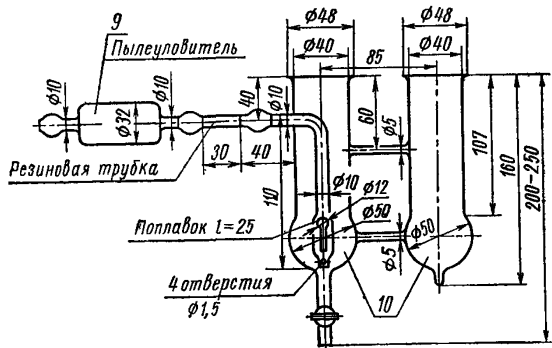
Черт.2. Адсорбционный аппарат для определения серы
