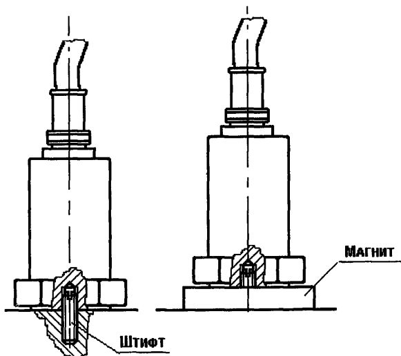
Рисунок 1 – Крепление датчика вибрации на опоре
