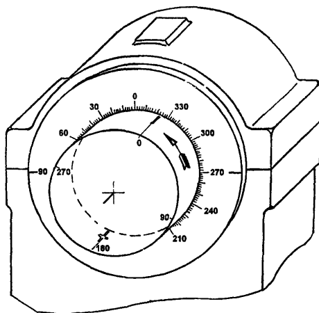
Рисунок 3 – Разметка ротора и статора агрегата при измерении фазы вибрации стробоскопическим способом
