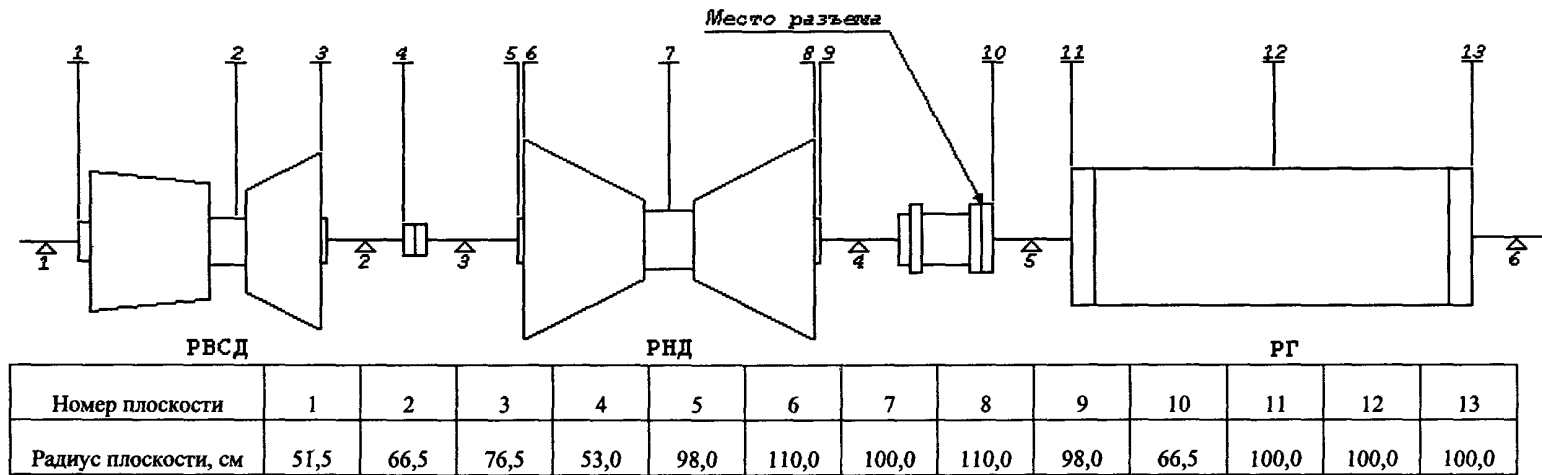
Рисунок 1.6 – Схема расположения плоскостей коррекции на турбоагрегате К-500-60/1500 ХТГЗ+ТГВ-500-4
