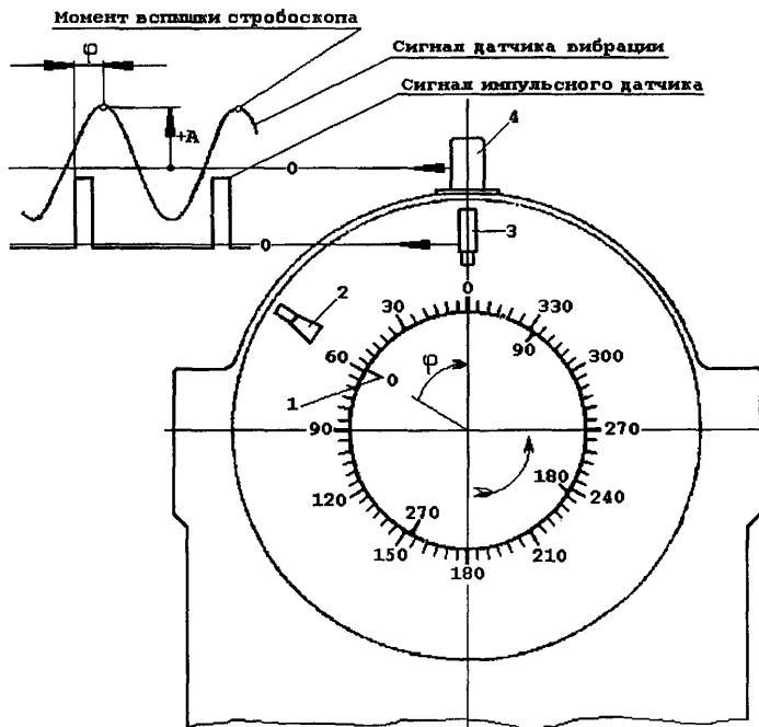
Рисунок 2 – Измерение фазы вибрации при балансировке
