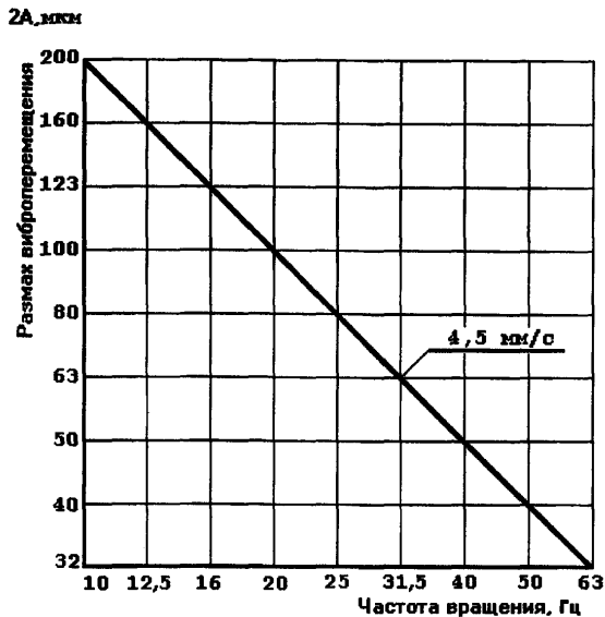
Рисунок 7 – График для определения допустимого размаха виброперемещения опор турбоагрегата на резонансных частотах
