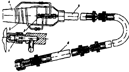
Рис. Ручная горелка:
