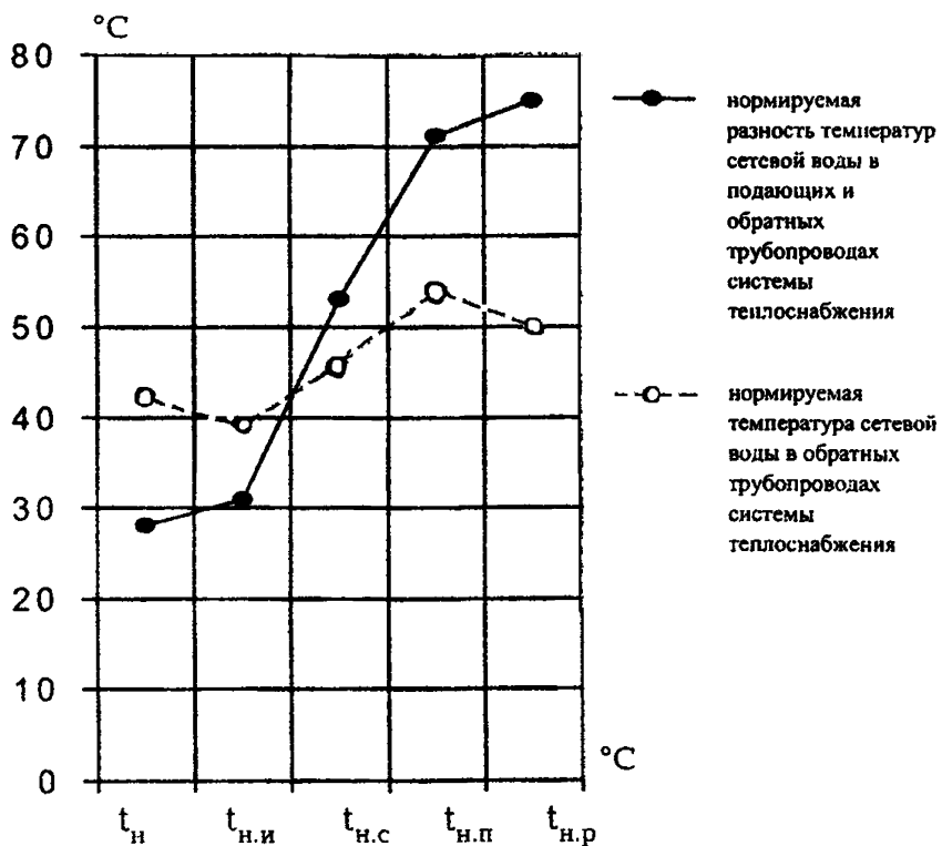
График изменения нормируемых разностей температур сетевой воды в подающих и обратных трубопроводах и температур обратных трубопроводов при характерных значениях температуры наружного воздуха
