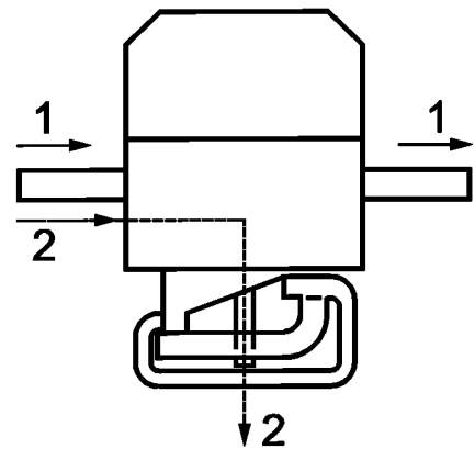
Рисунок 4 — Испытание на тепловой ток короткого замыкания
