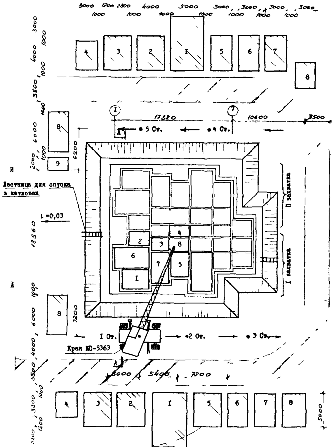
Рис. I. Схема организации работ при монтаже скользящей опалубки
