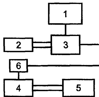
1 — вольтметр; 2 — осциллограф; 3 — аппарат «Нэйва-2к»; 4 — устройство измерения давления; 5 — импульсный генератор МИГ-1к; 6 — датчик давления Т-2000
