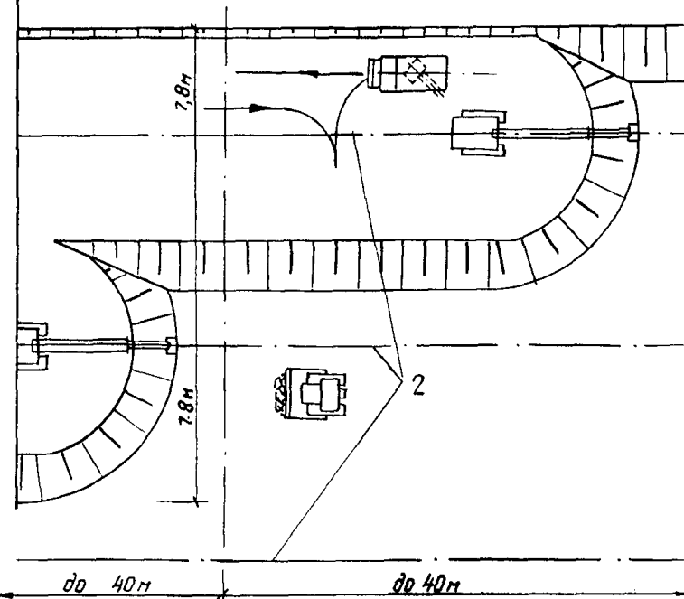
План потока
