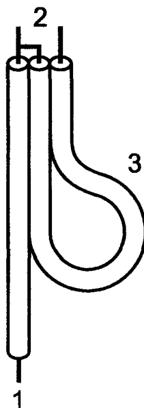
1 — несимметричный вход; 2 — симметричный выход; 3 — полуволновая петля
