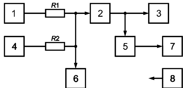
1 — генератор сигналов НЧ; 2 — передатчик; 3 — эквивалент антенны; 4 — генератор сигналов НЧ; 5 — элемент связи; 6 — милливольтметр НЧ; 7 — модулометр; 8 — анализатор спектра ВЧ; R_1 , R_2 — резисторы сопротивлением (6,8 \pm 0,34) кОм
