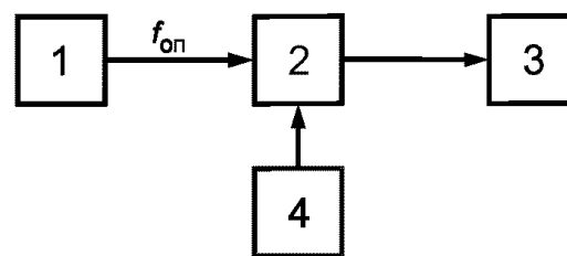
1 — возбuditель передатчика; 2 — частотный компаратор; 3 — частотомер; 4 — стандарт частоты; f_{оп} — опорная частота
